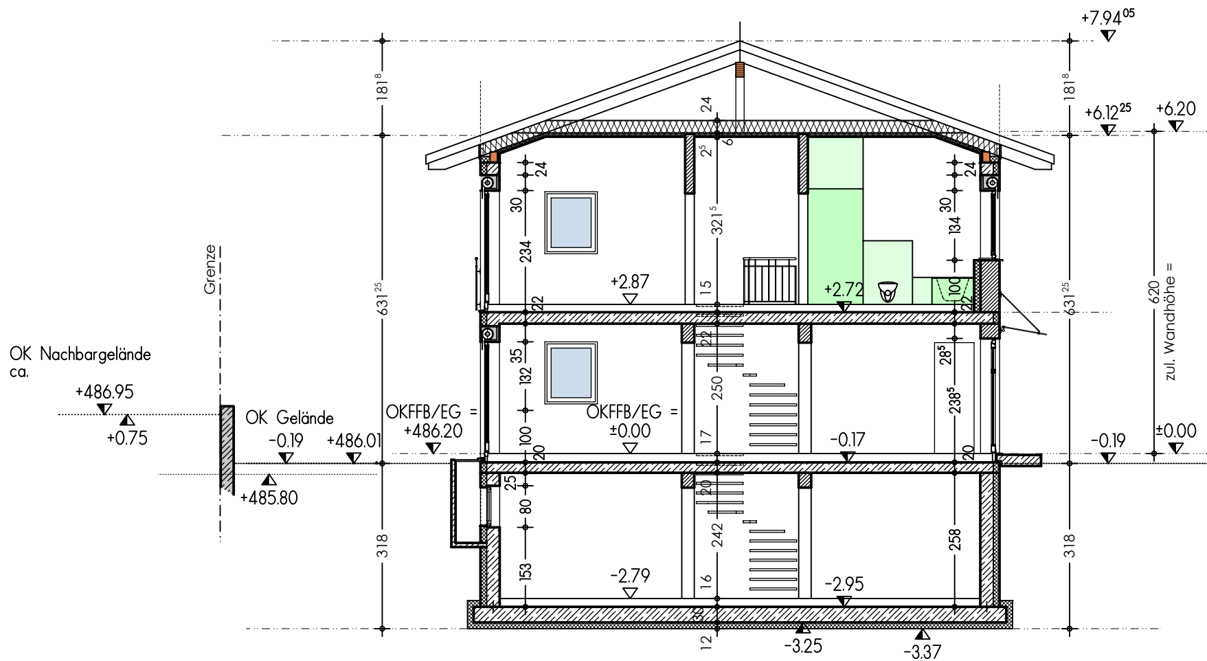
DH * SCHNITT 1 - 1
