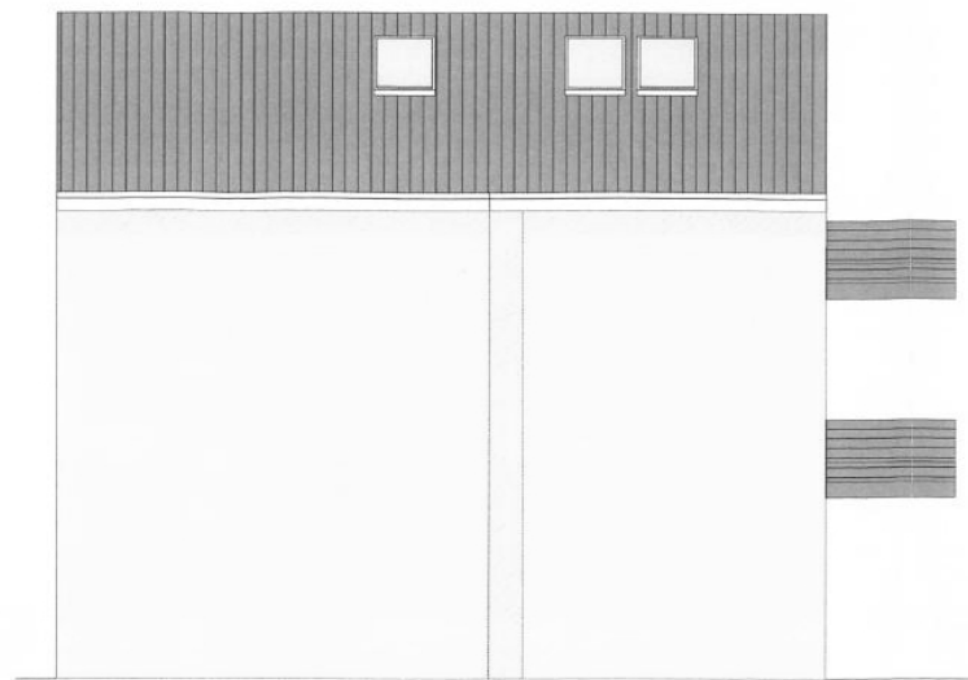
NORD-WEST-ANSICHT
