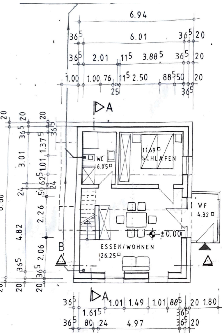
GRUNDRISS ERDGESCHOSS „FERIENWOHNUNG“
