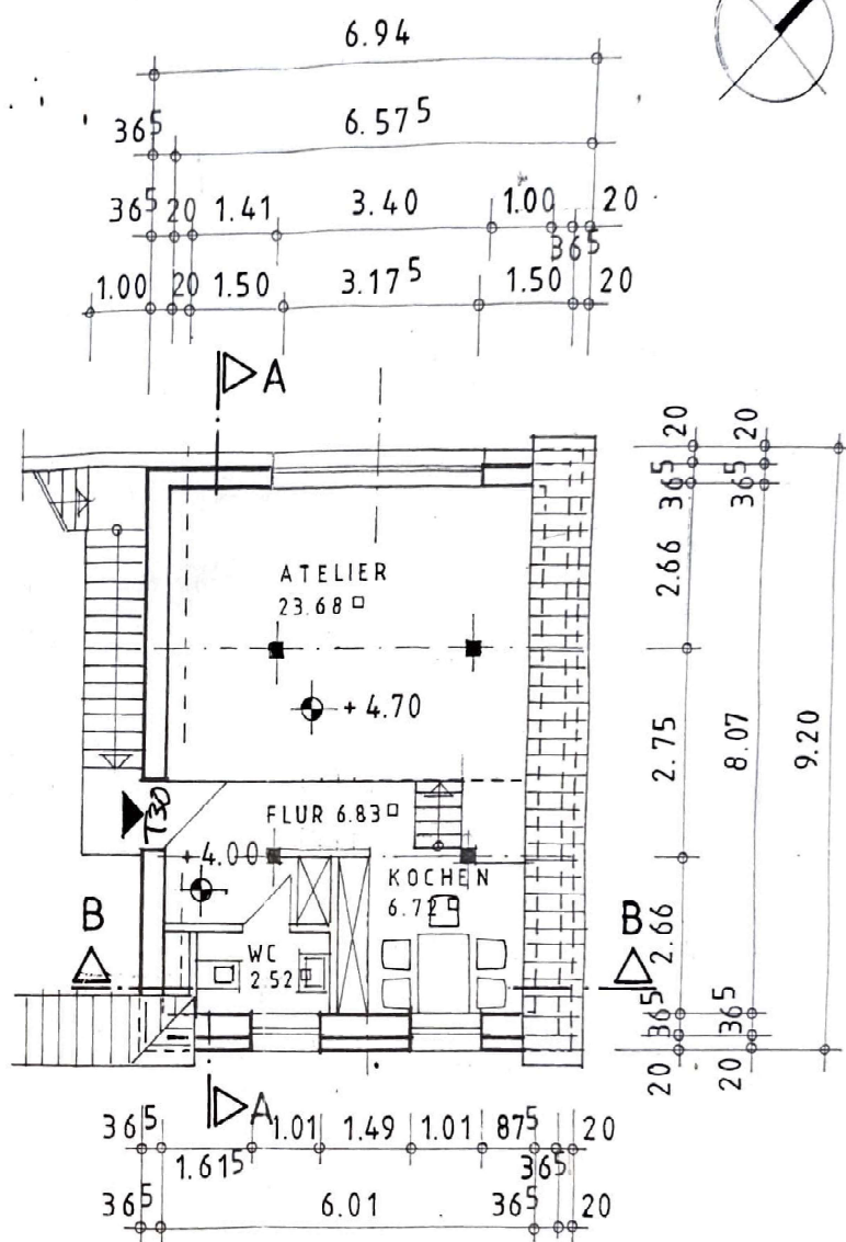
GUNDRISS DACHGESCHOSS „ATELIER“
