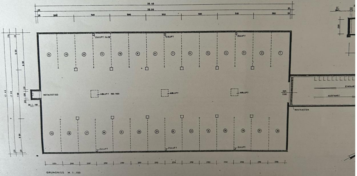
GRUNDRISS M 1:100
