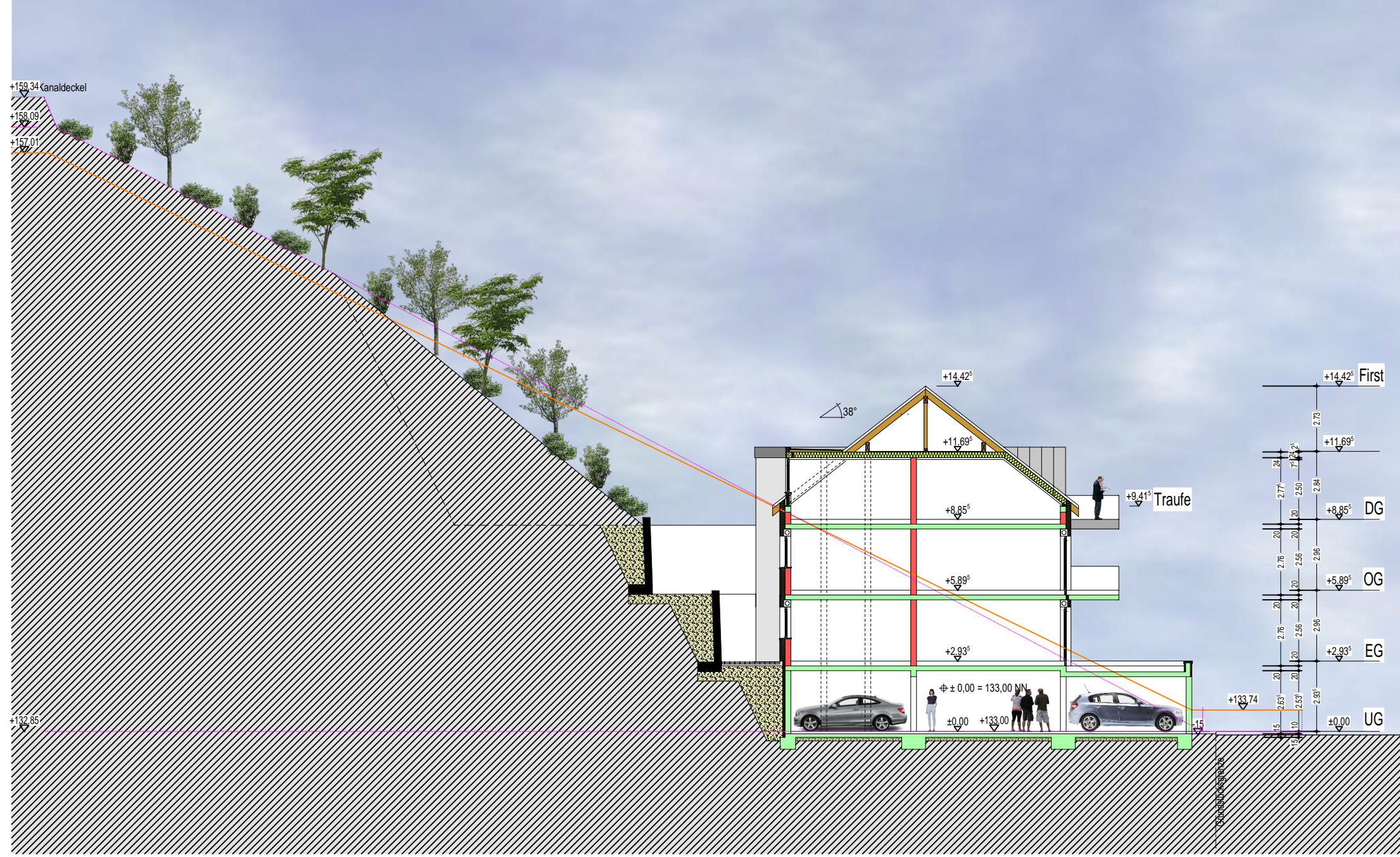
SYSTEMSCHNITT
