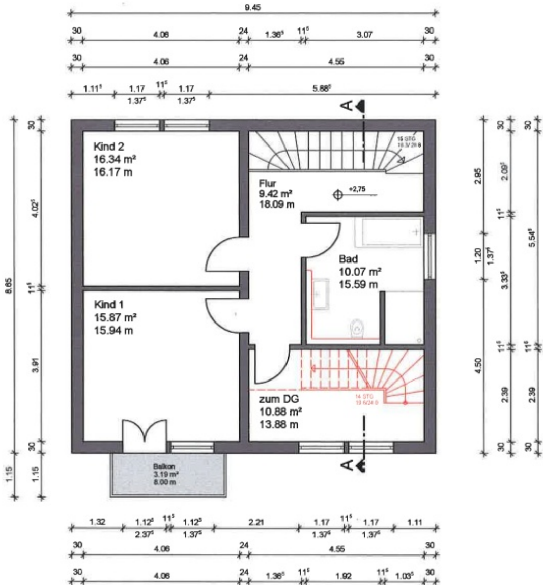
GRUNDRISS OBERGESCHOSS
