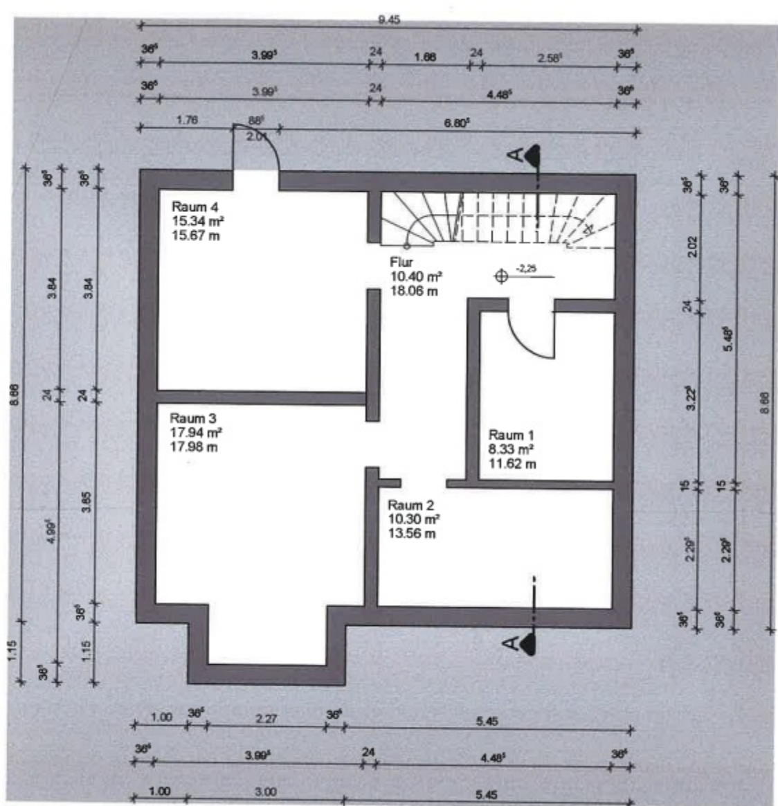
GRUNDRISS KELLERGESCHOSS
