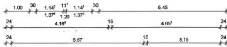
GRUNDRISS DACHGESCHOSS
