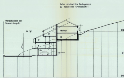
SCHNITT 4
