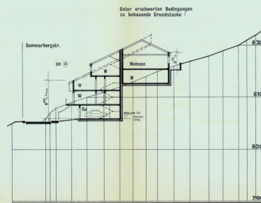
SCHNITT 3
