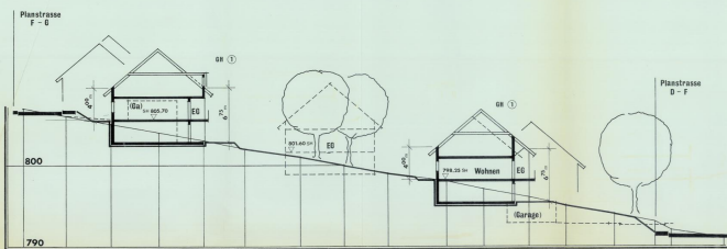
SCHNITT 1
