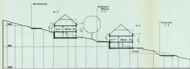
SCHNITT 2
