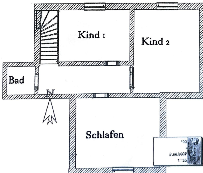
OG Grundrissplan ohne Maßstab
