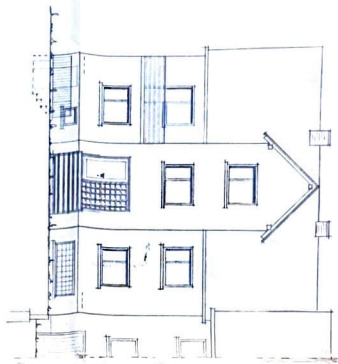
NORD-WEST ANSICHT
