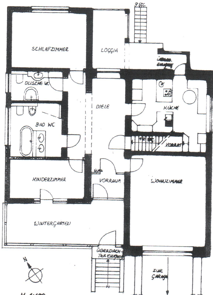
M 1:100 ERDGESCHOSS
