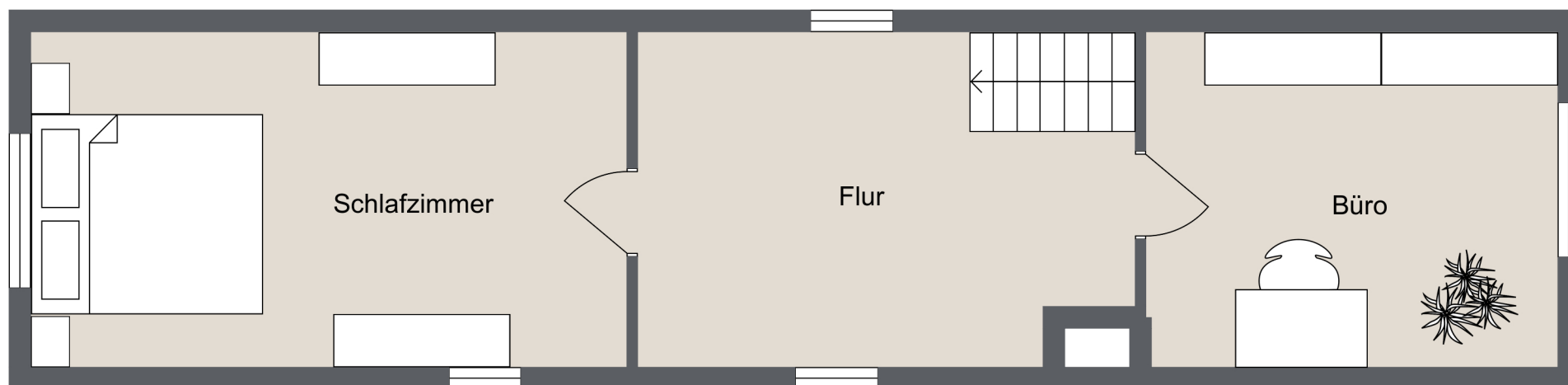
Dachgeschoss
