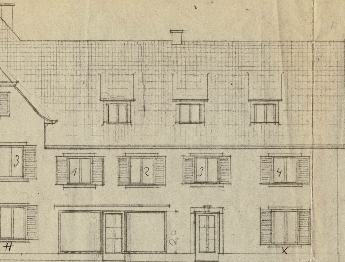
STRASSEN-ANSICHT
