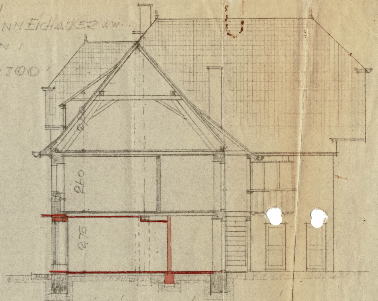
SCHNITT AB - MIT SEITENANSICHT
