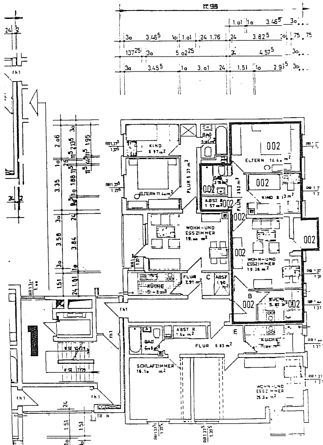
Wohnung 002
