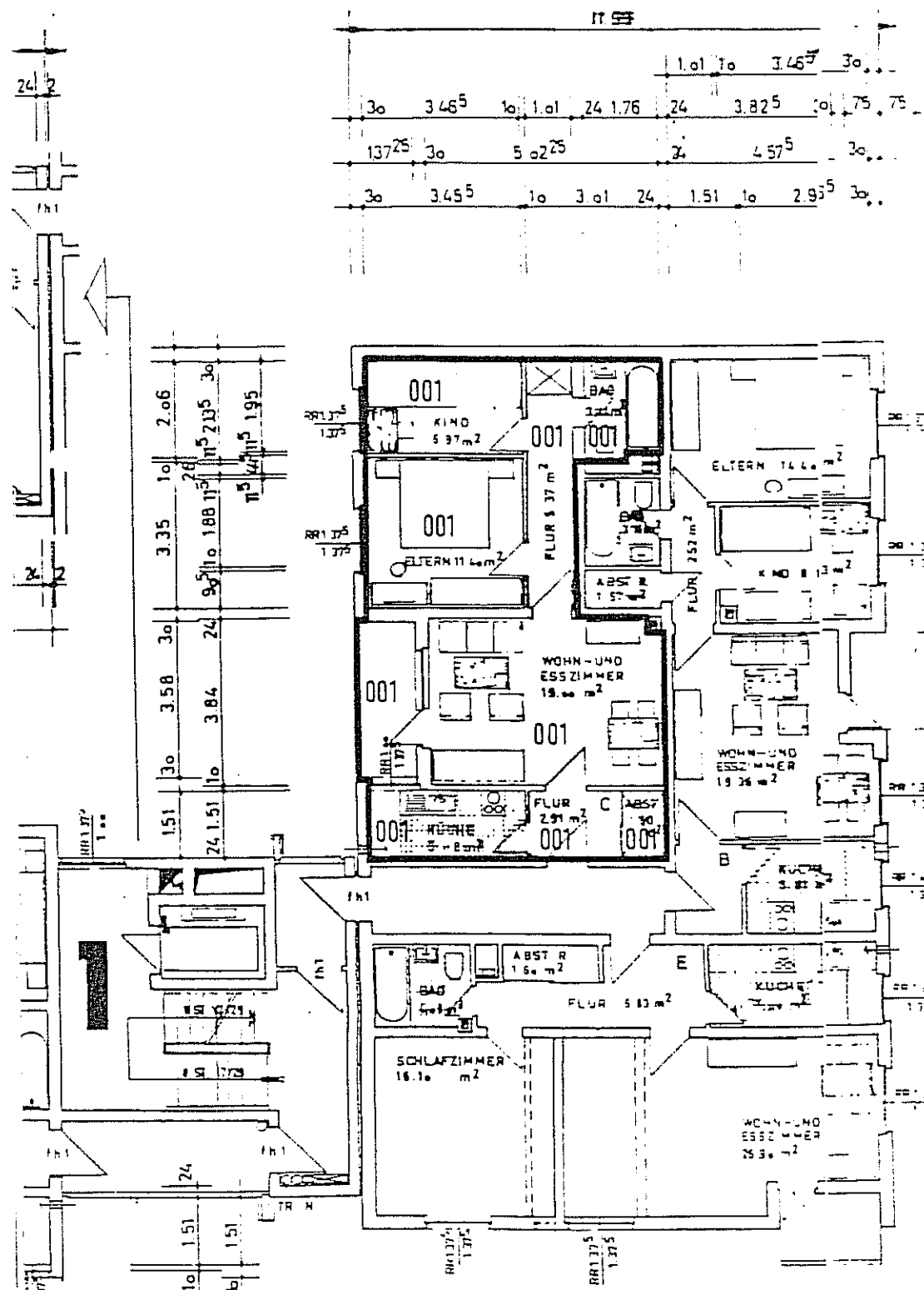
Wohnung 001
