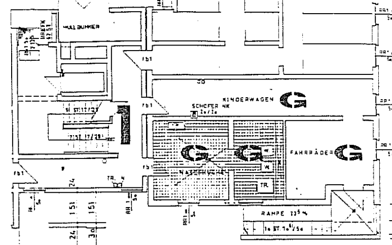
GEMEINSCHAFTSRÄUME KG.
