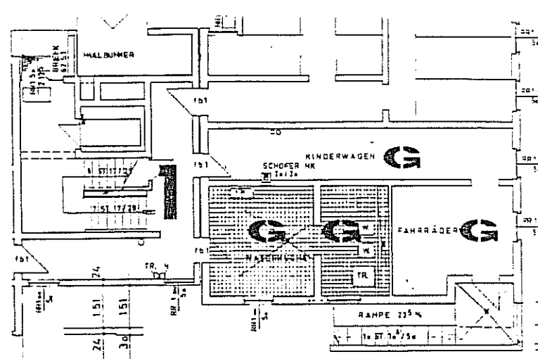
GEMEINSCHAFTSRÄUME KG. GEMEINSCHAFTSRÄUME 11.06.
