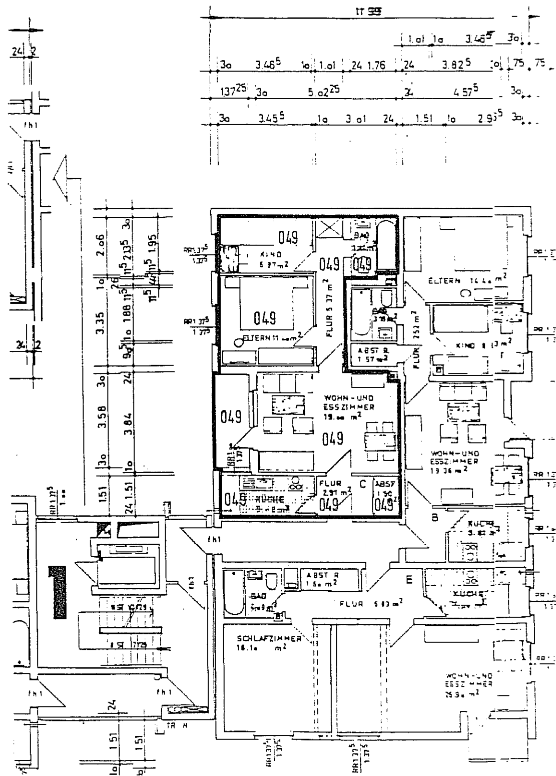
Wohnung 049
