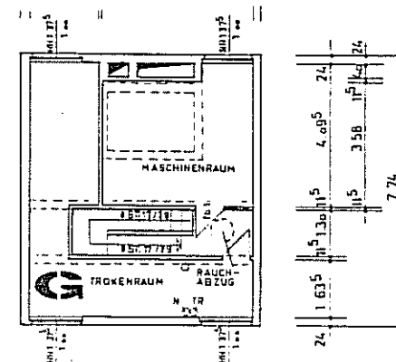
GEMEINSCHAFTSRÄUME KG. GEMEINSCHAFTSRÄUME 11.06.
