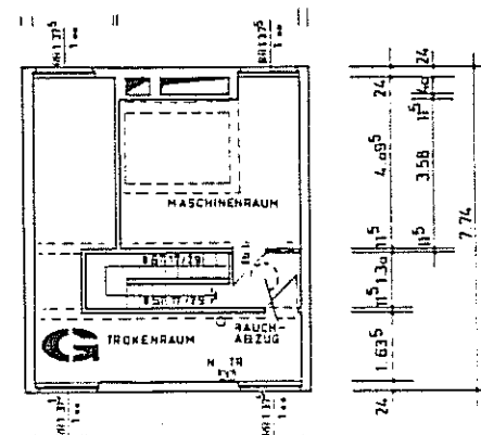
GEMEINSCHAFTSRÄUME KG. GEMEINSCHAFTSRÄUME 11. OG.
