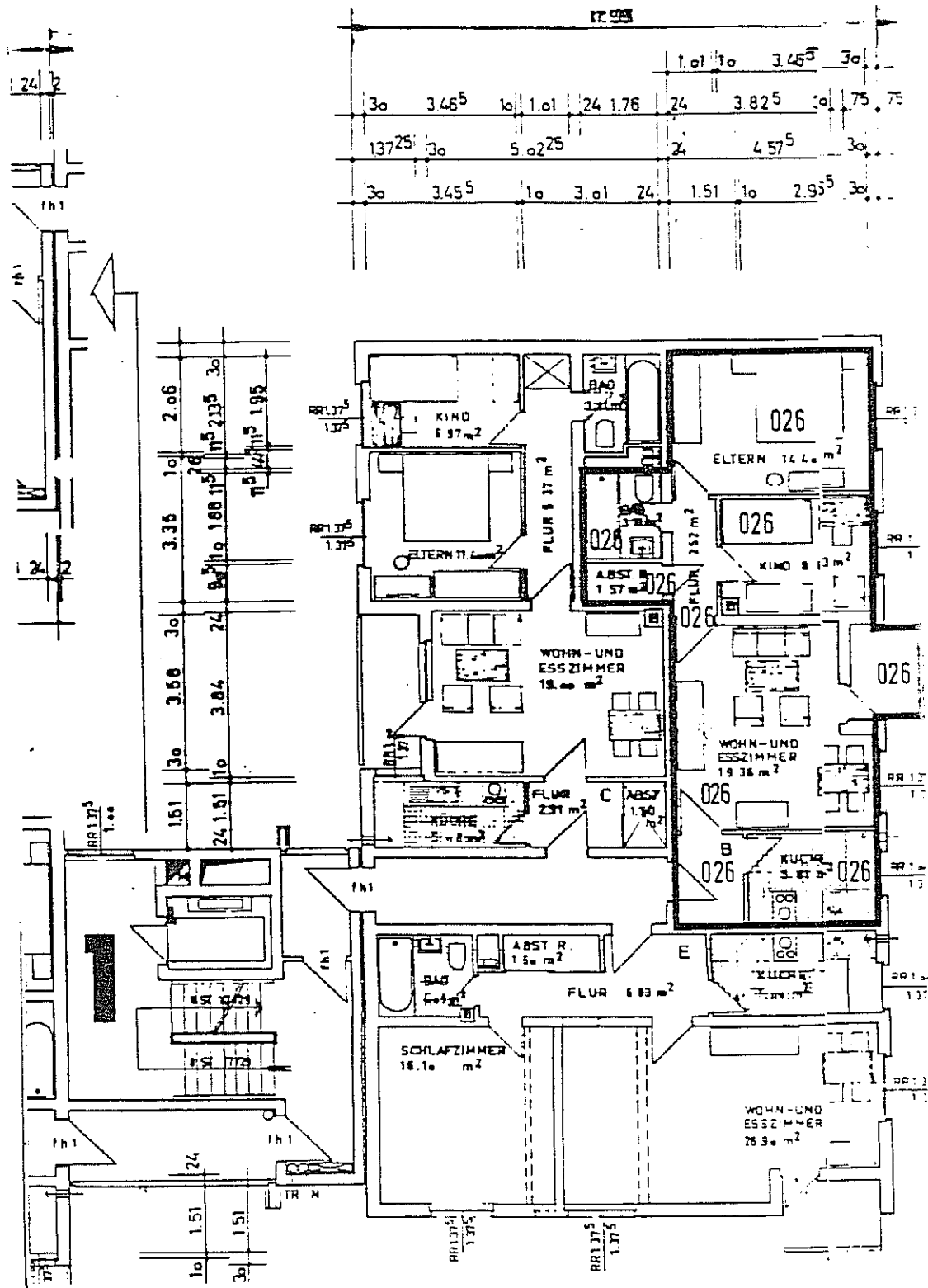
Wohnung 026
