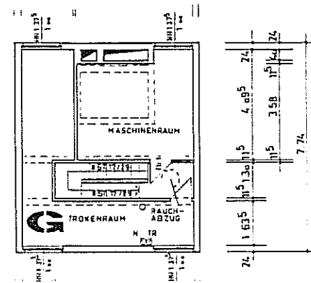
GEMEINSCHAFTSRÄUME 11.06.
