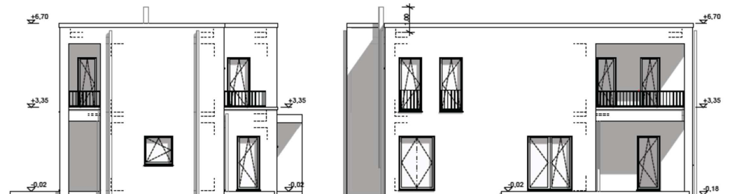
Ansicht Ost
