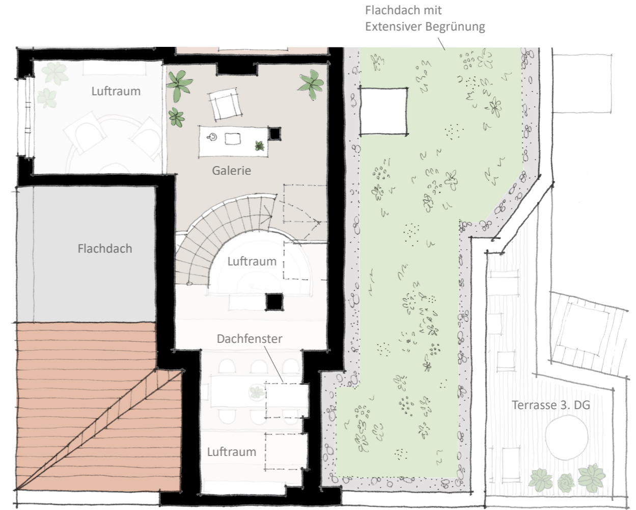
Grundriss 4. DG
