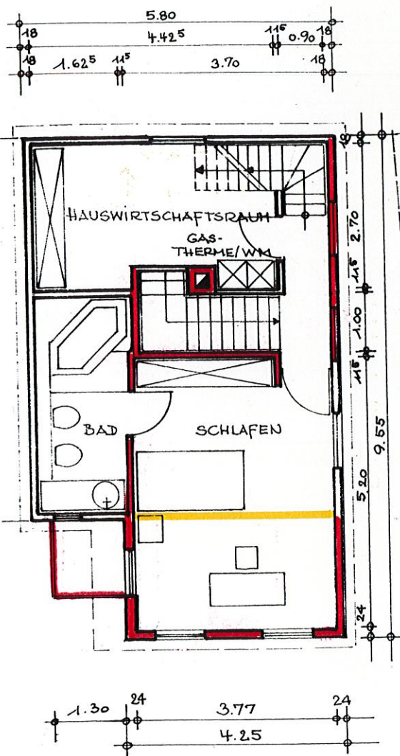
OBERGESCHOSS
