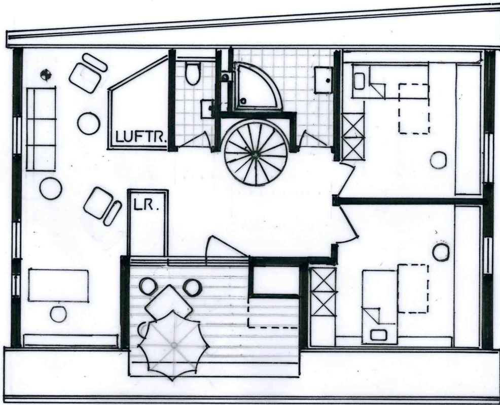
DACHGESCHOSS
