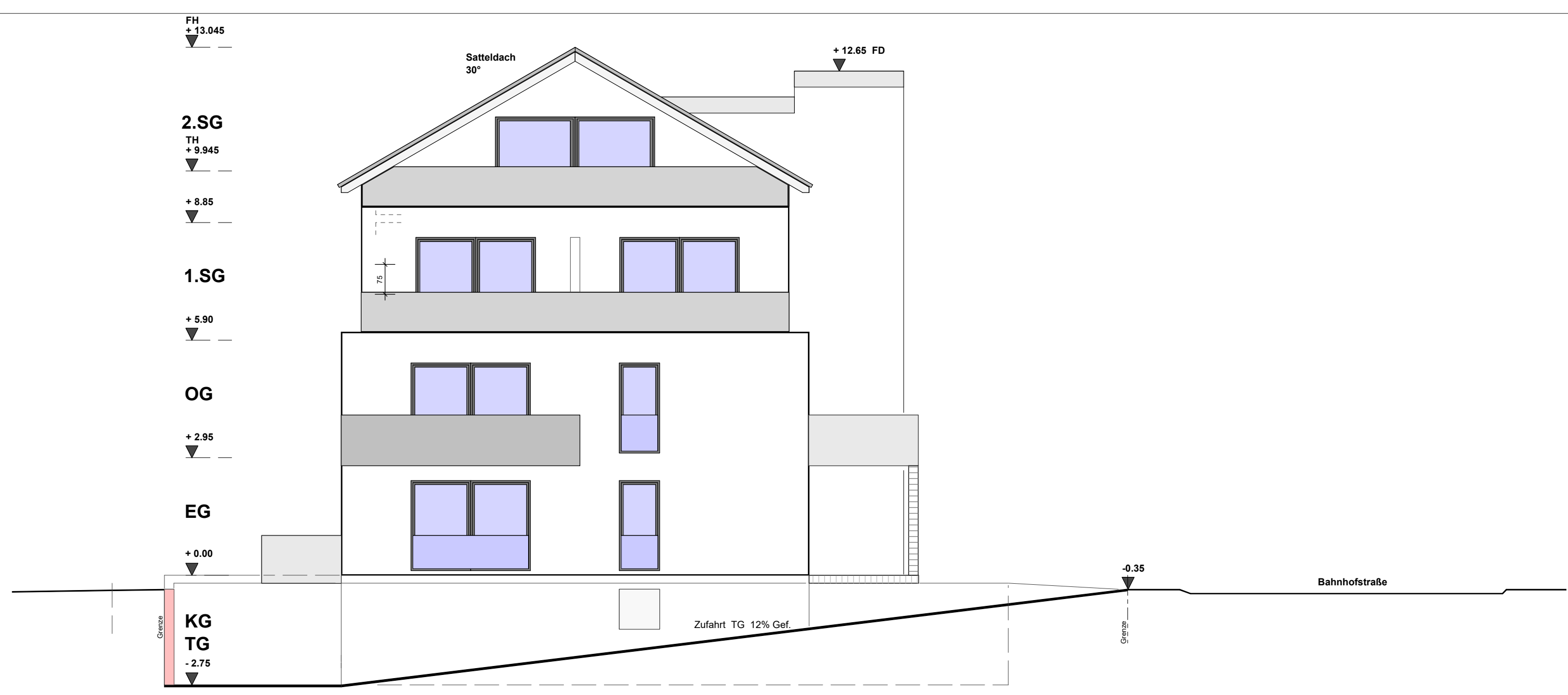
West-Ansicht
