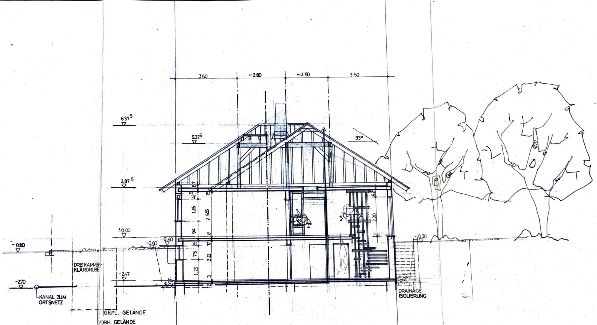
SCHNITT + ENTWÄSSERUNG + QUERPROFIL
