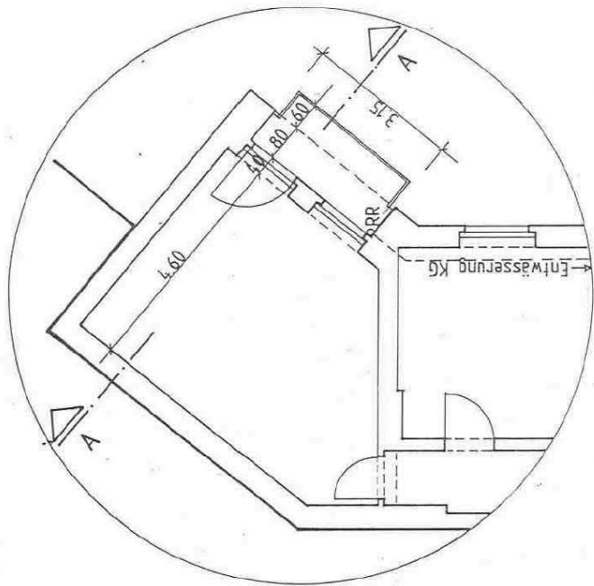
AUSSCHNITT GRUNDRISS 1:100
