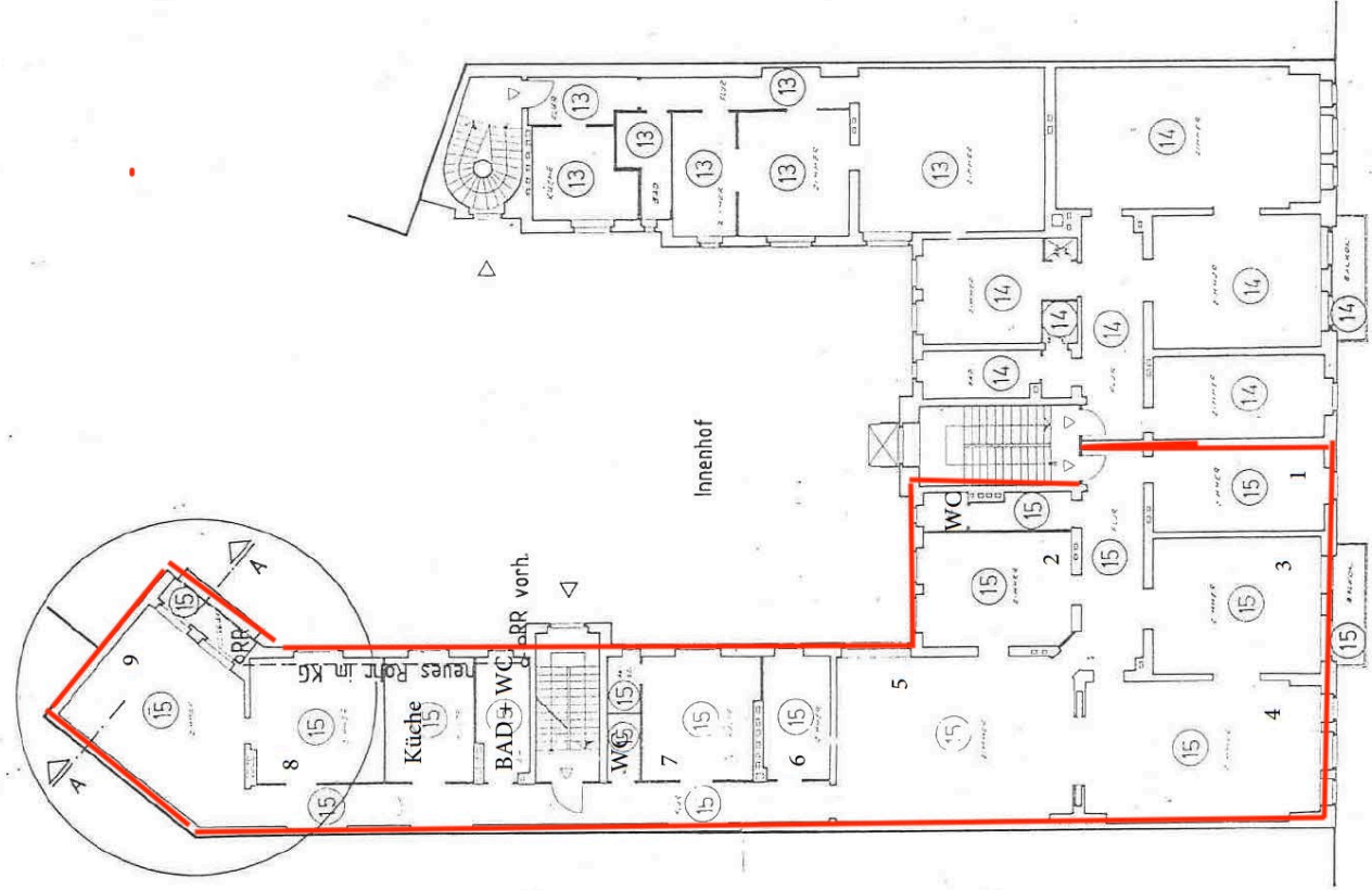
AUSSCHNITT GRUNDRISS 1:100
