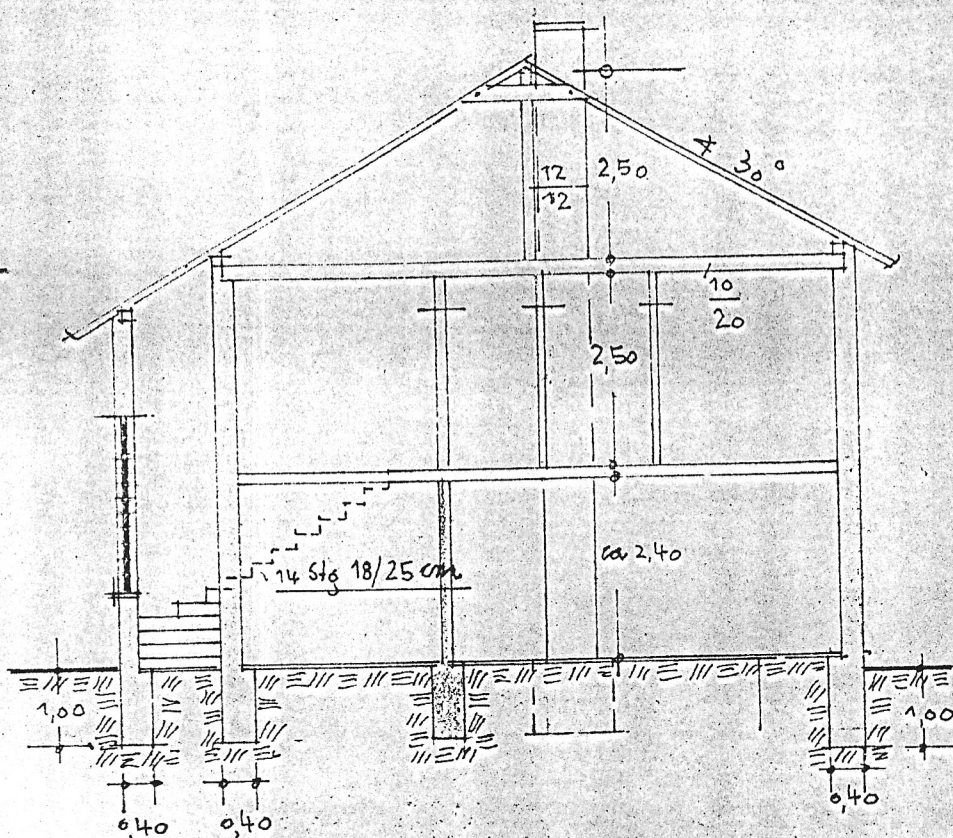
SNITT A-B
