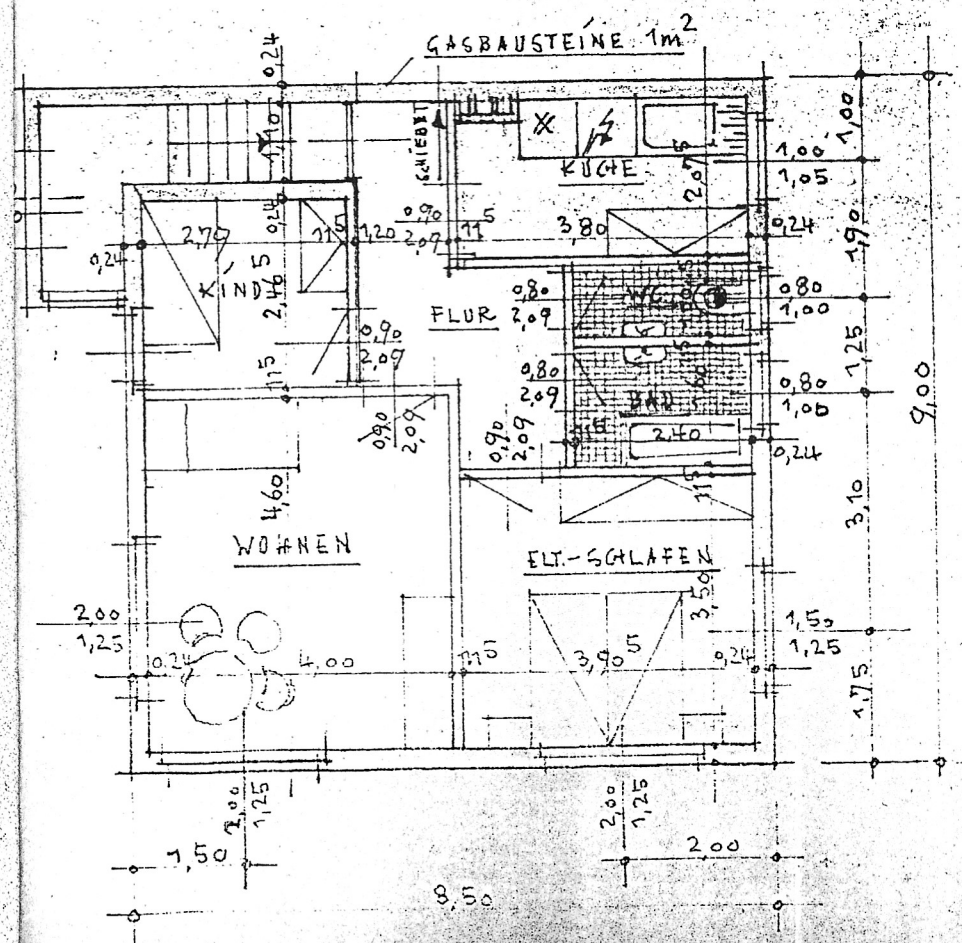
OBERGESCHOSS
