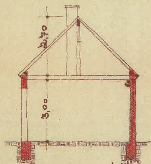
QUERSCHNITT A-B
