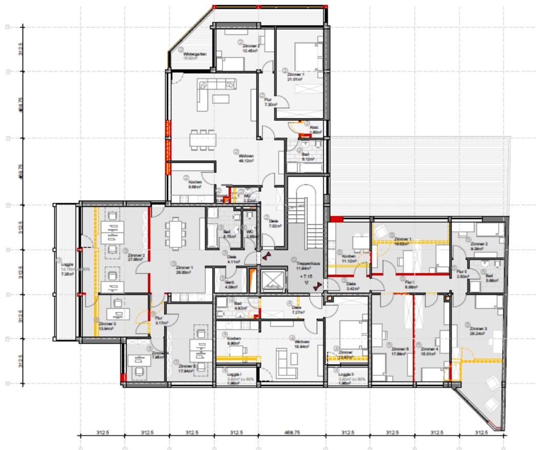
Grundriss Etage 2
