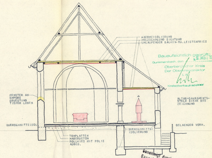
QUERSCHNITT MIT BLICK ZUR ALTARKONCH
