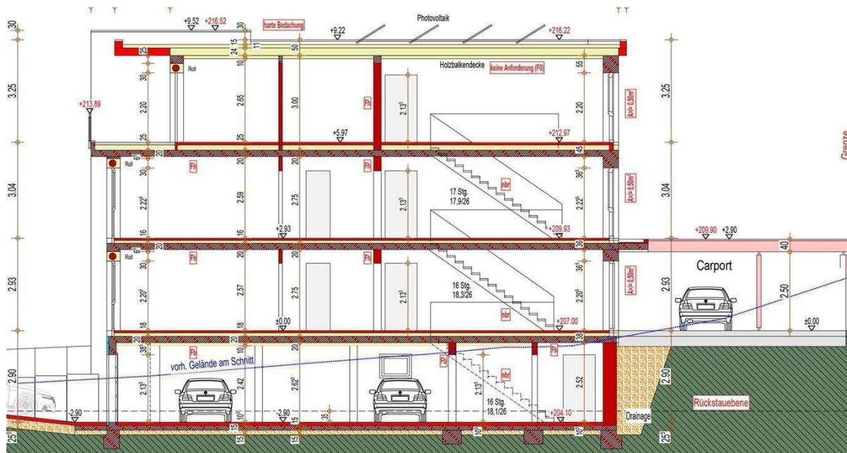
Gebäudeschnitt. Lift und Tiefgarage im Haus
