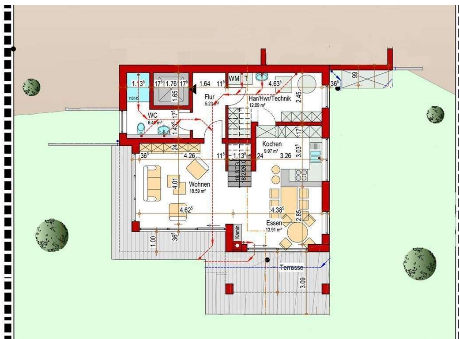
geplantes UG: 66,2 m 2 Wohnfläche mit großer Terrasse
