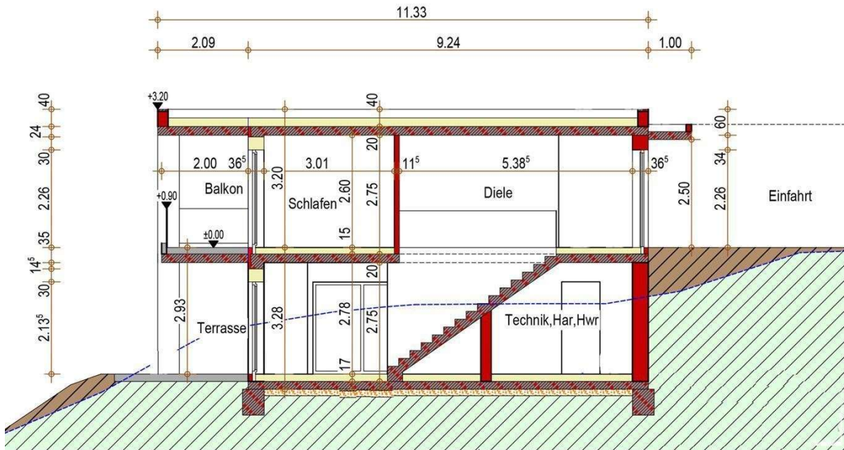
Schnittzeichnung Bungalow (Süd-Ost)
