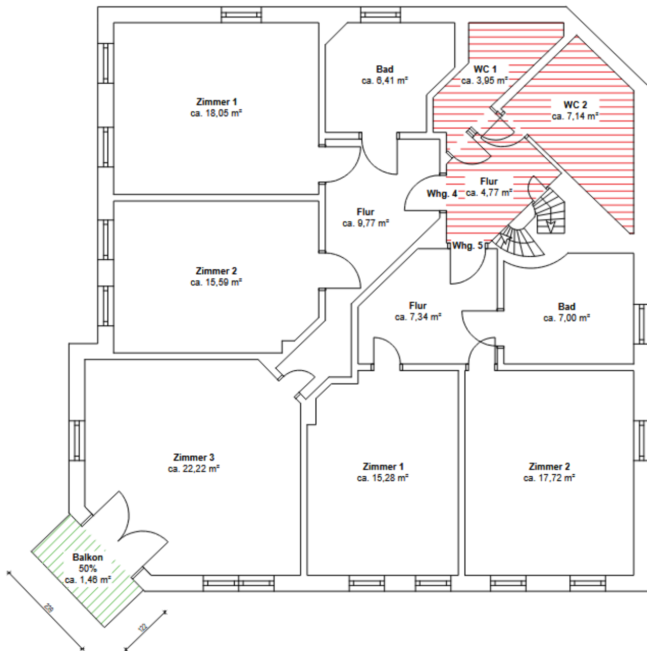
Grundriss 2. OG
