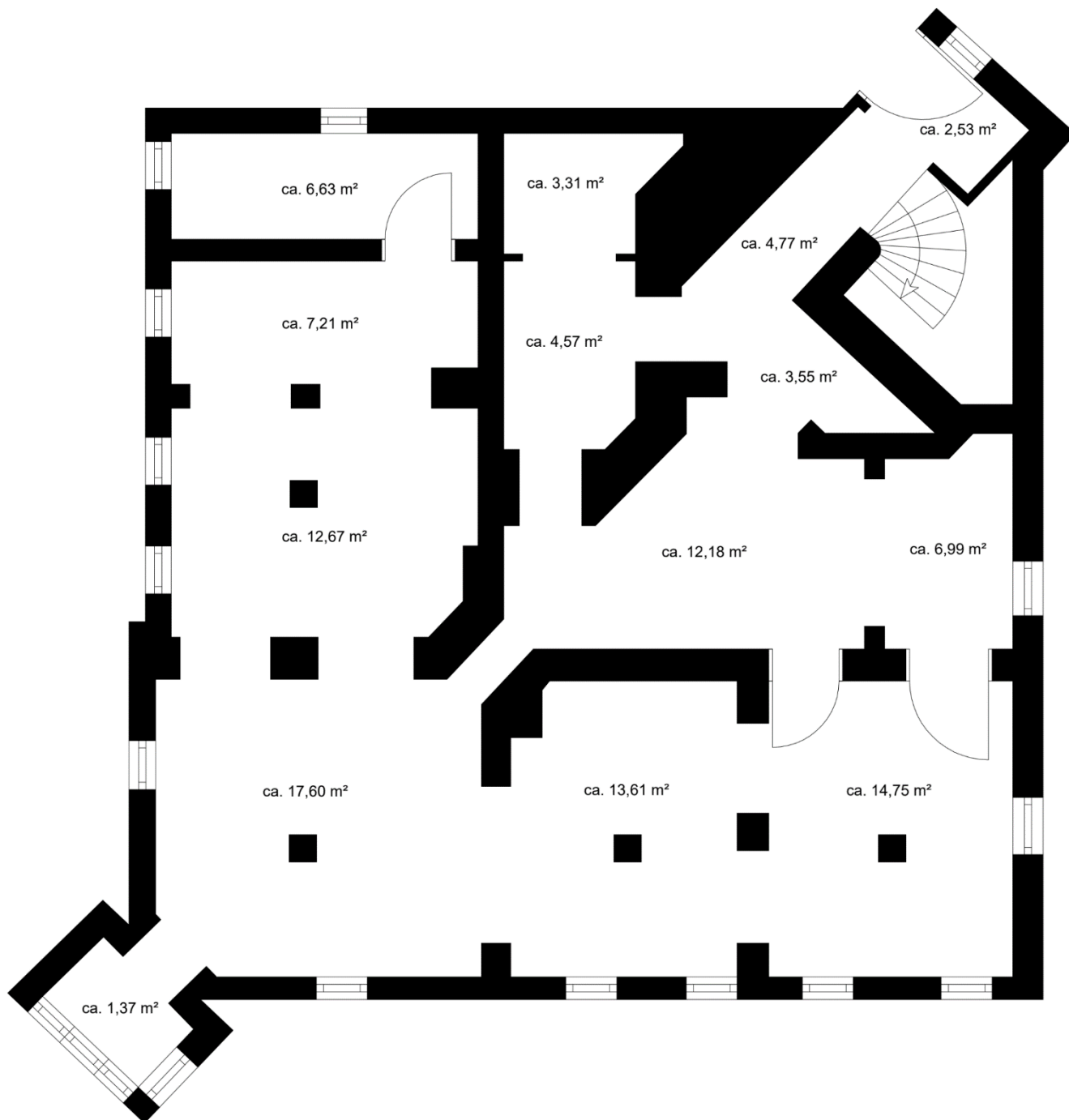
Grundriss KG
