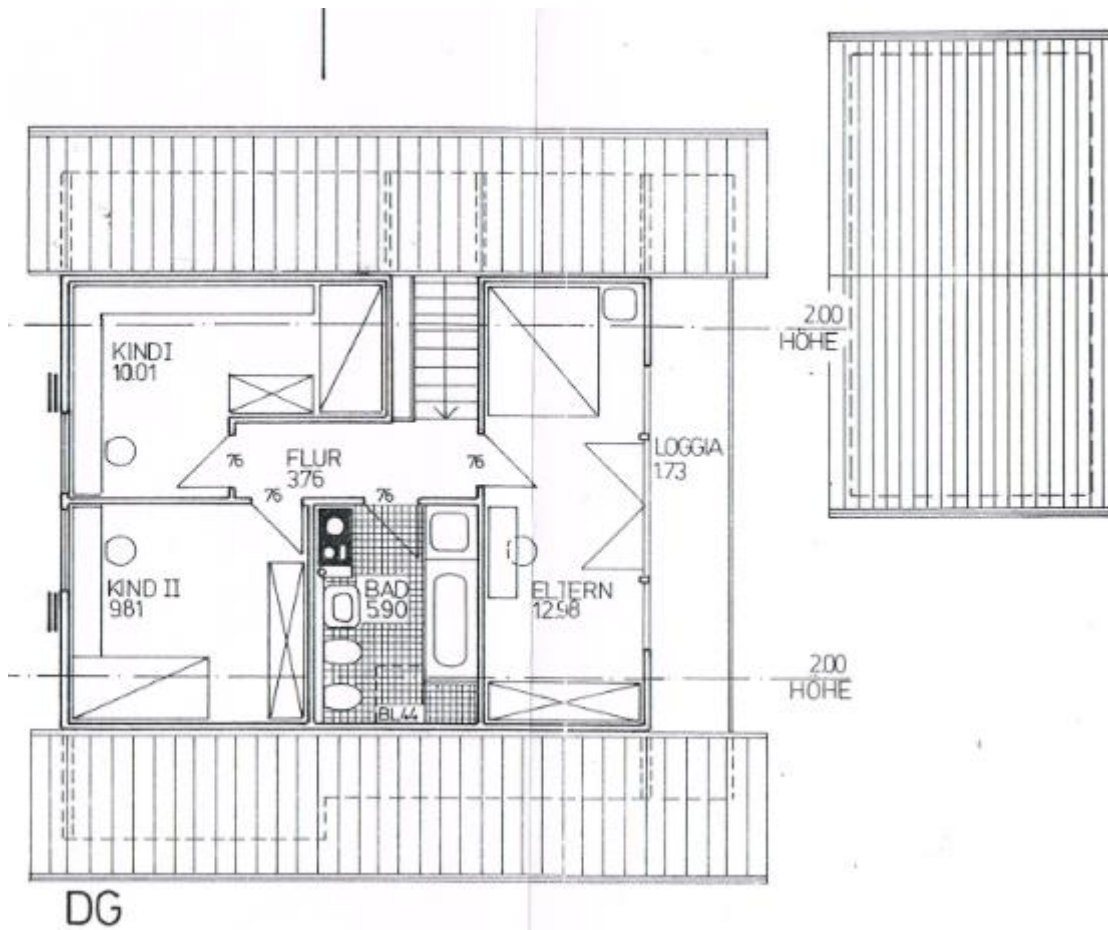
Grundriss DG
