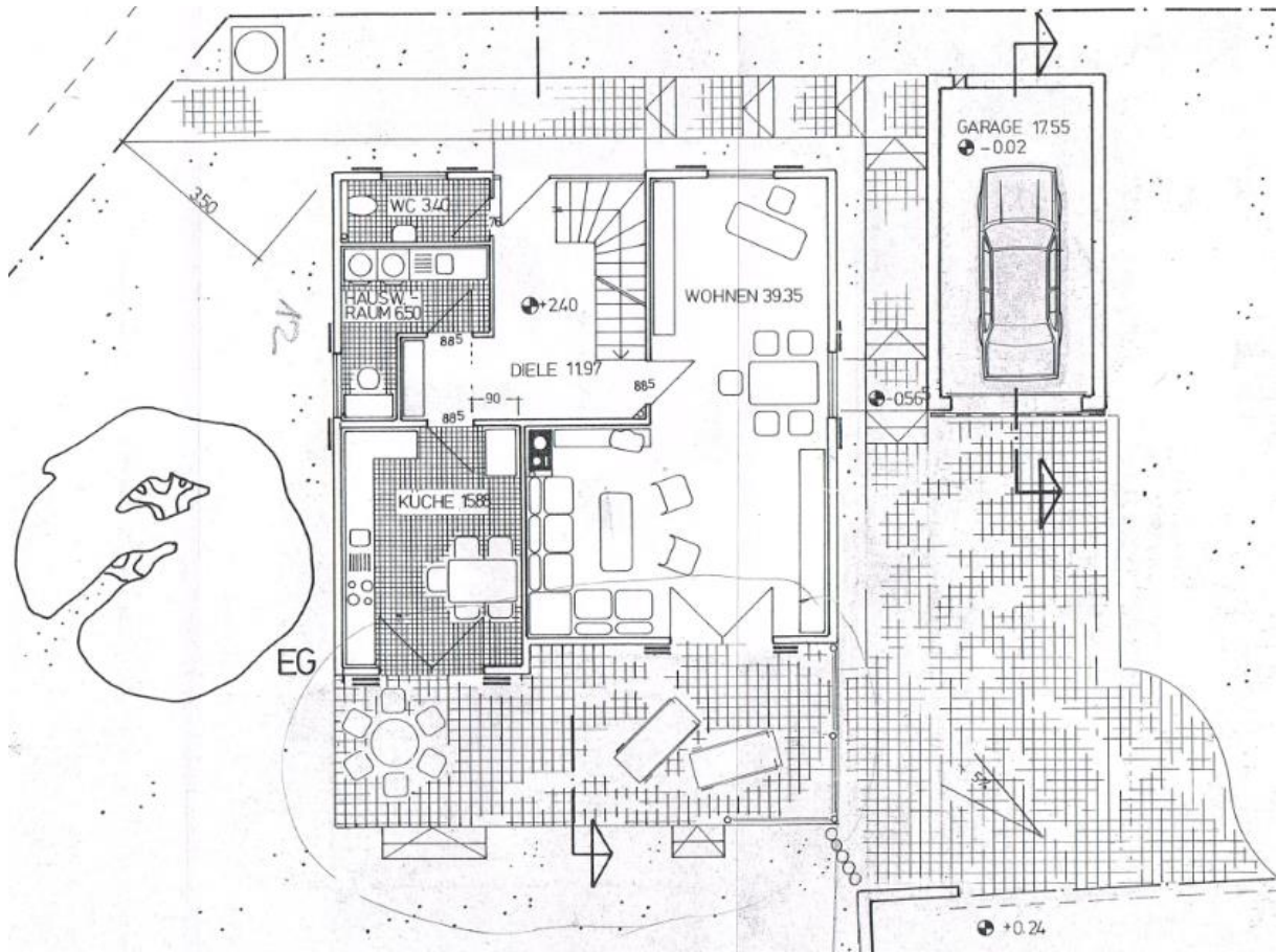
Grundriss EG
