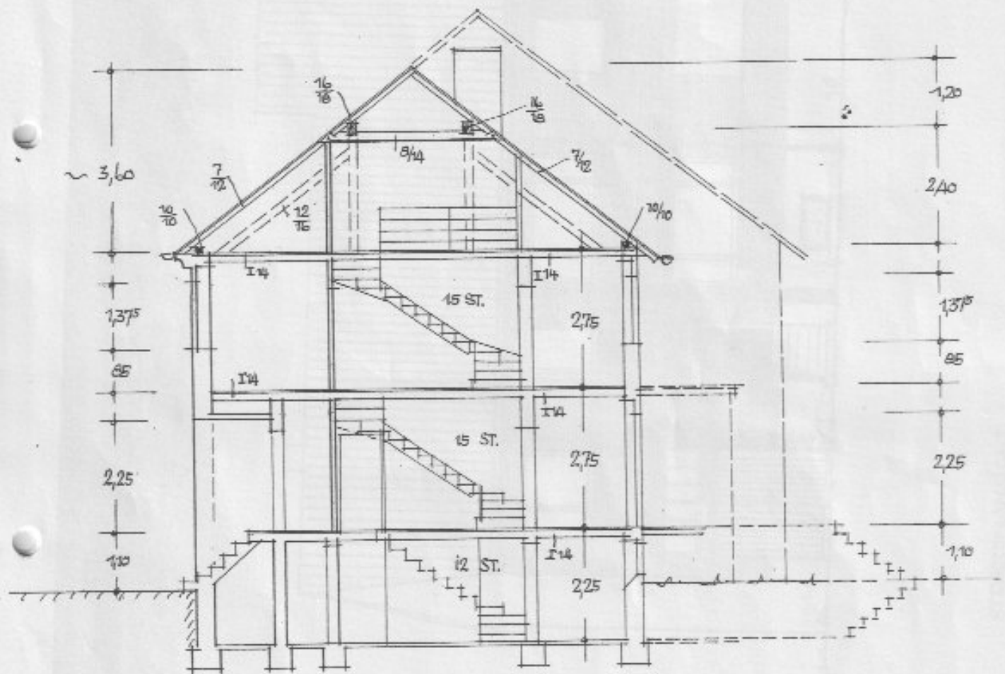
QUERSCHNITT
