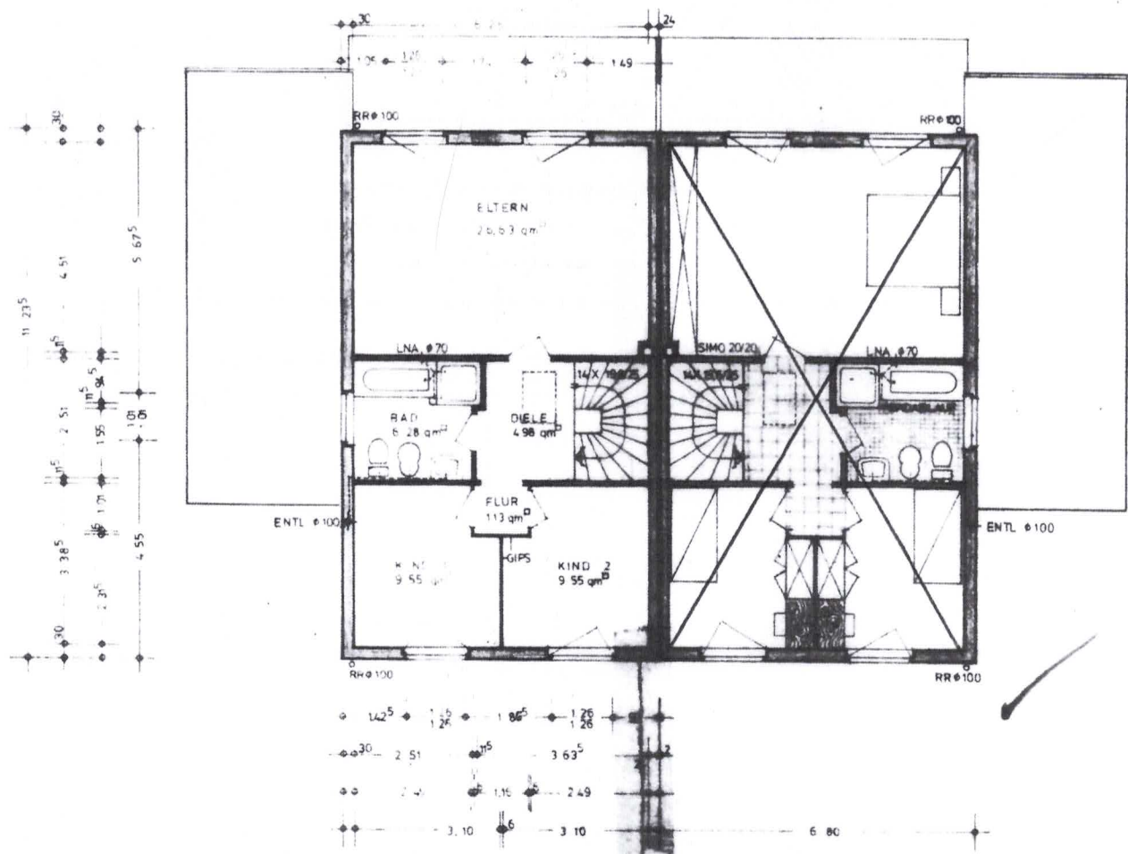
DACHGESCHOSS
