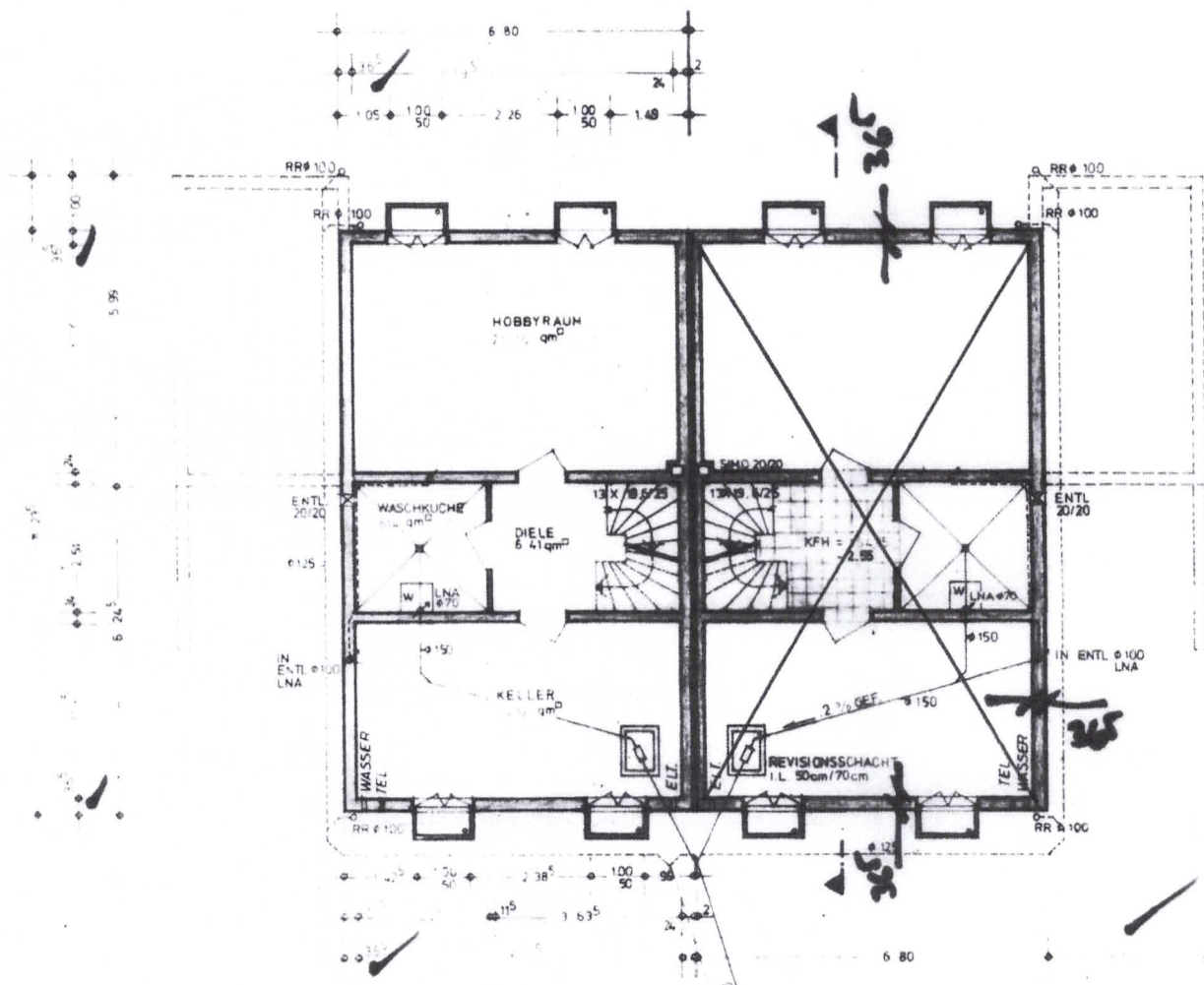
KELLERGESCHOSS
