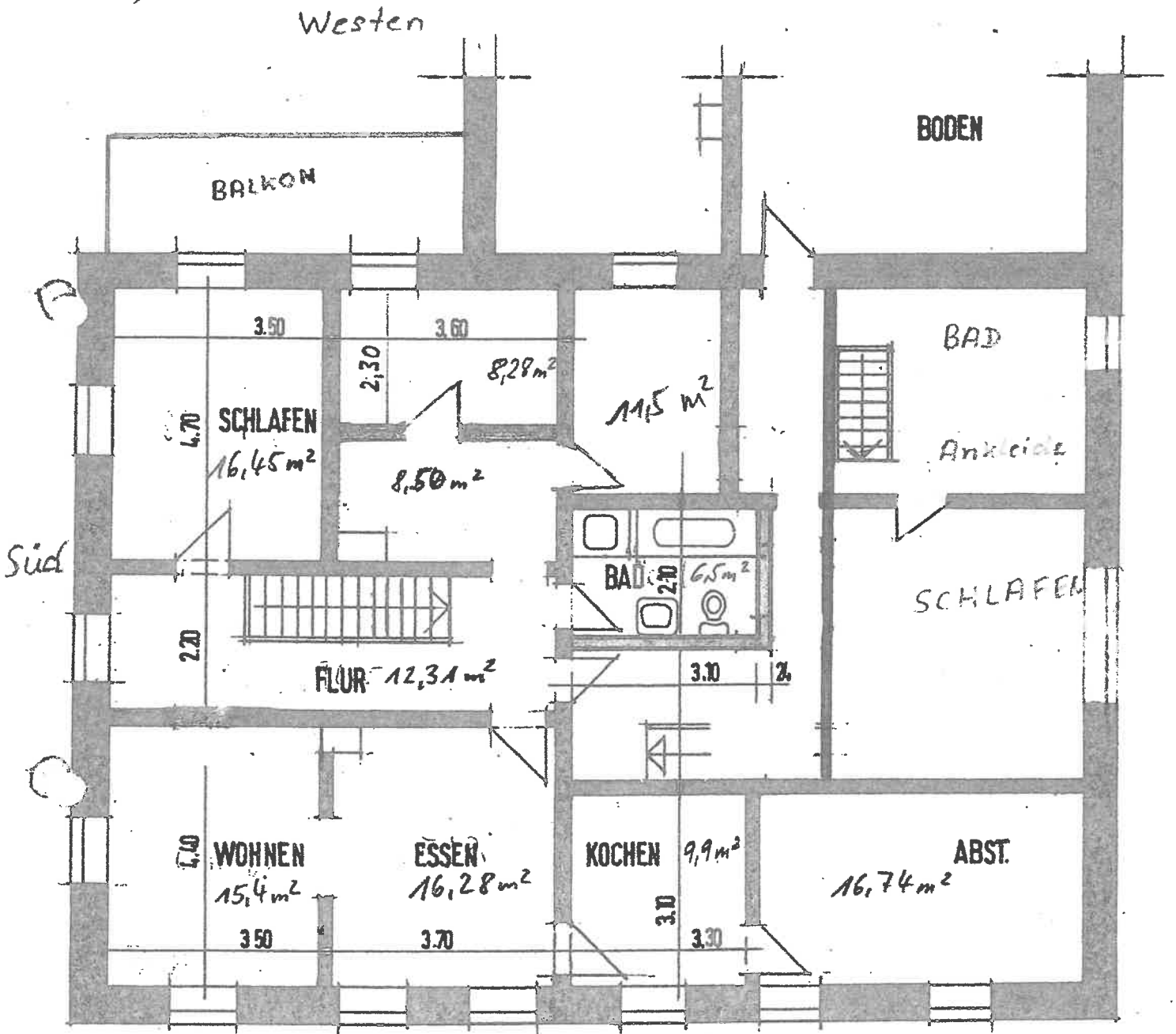
OBERGESCHOSS M.1:100
