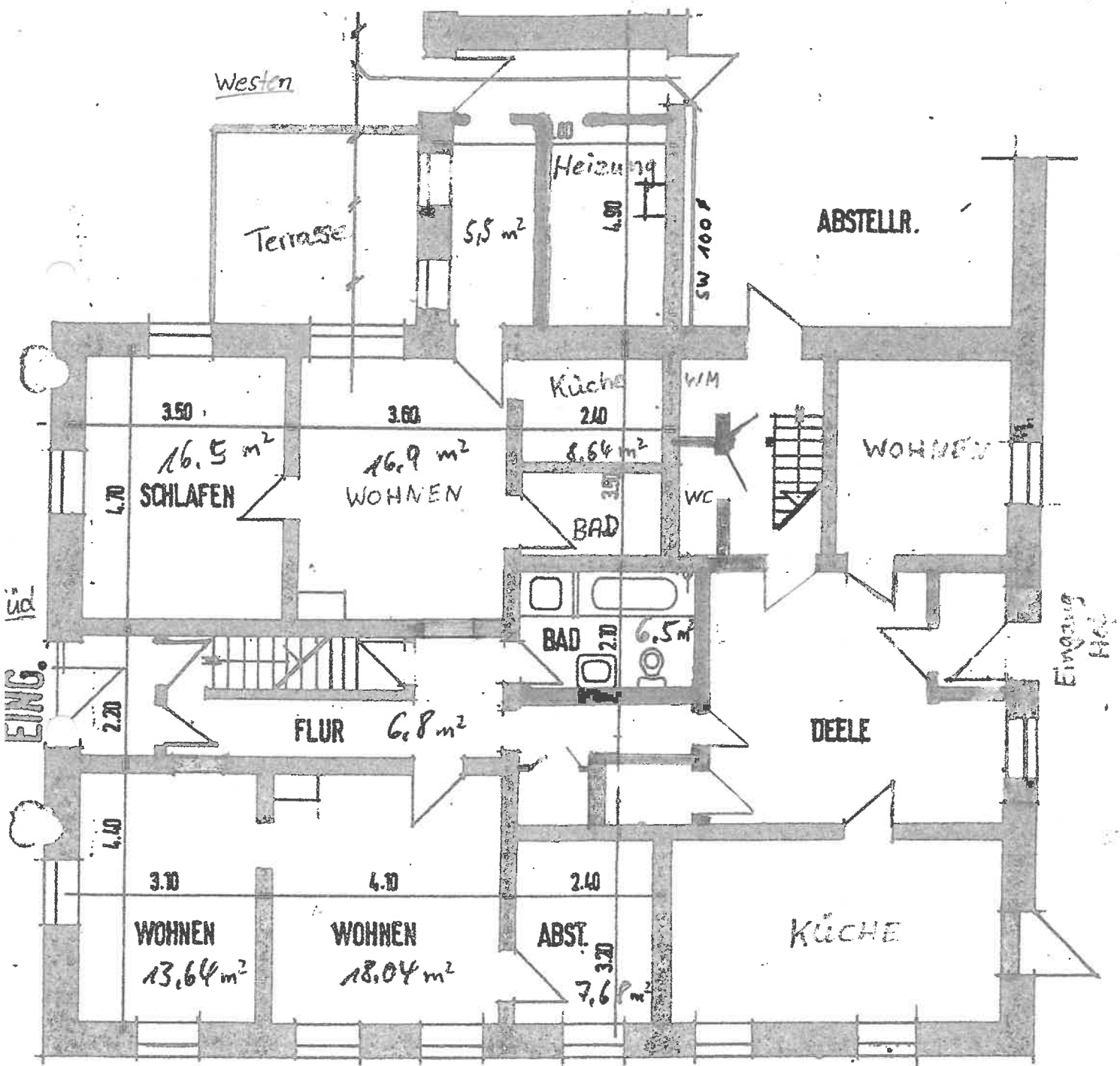
ERDGESCHOSS M.1:100
