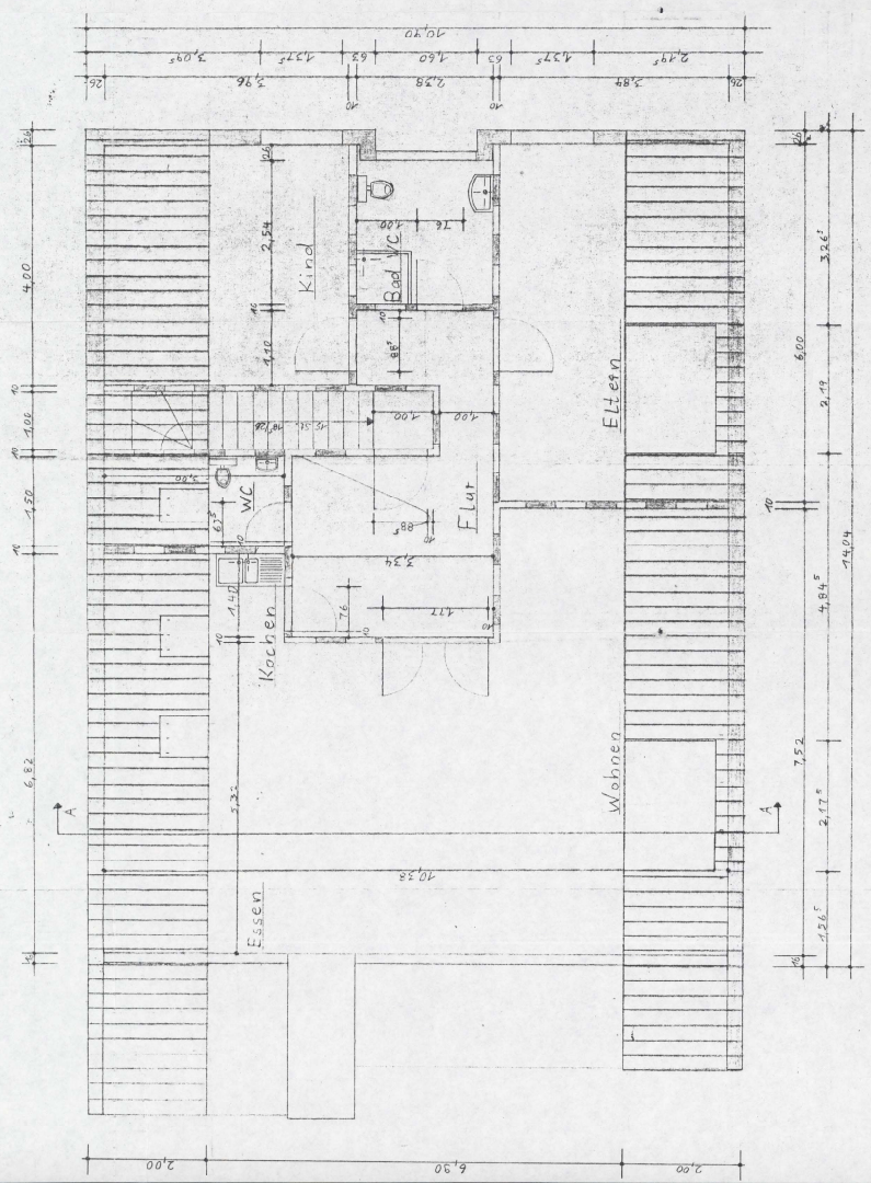
Dachgeschoss M 1:50
