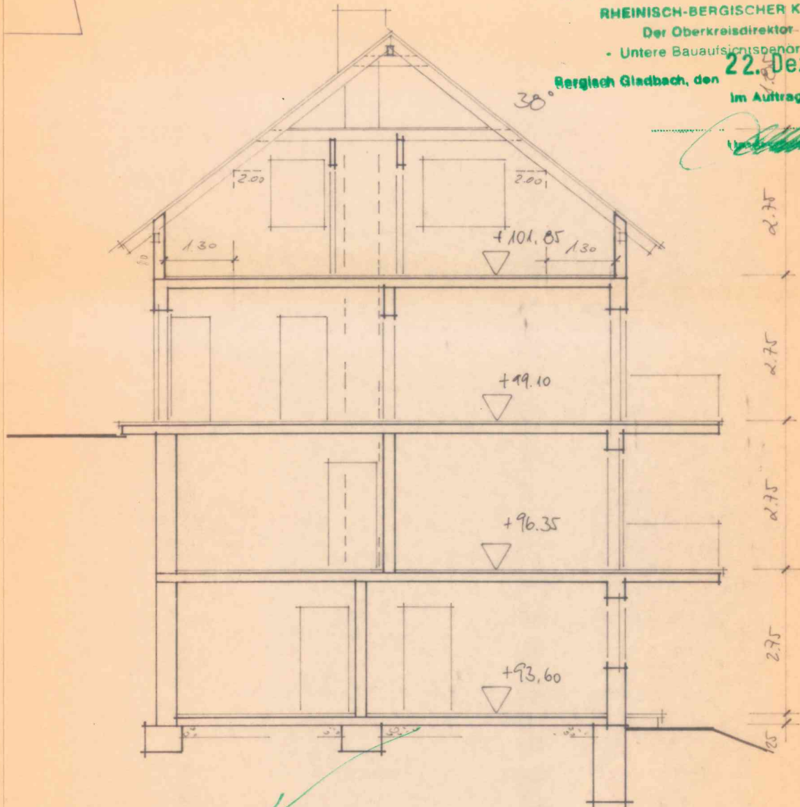
QUERSCHNITT A-B
