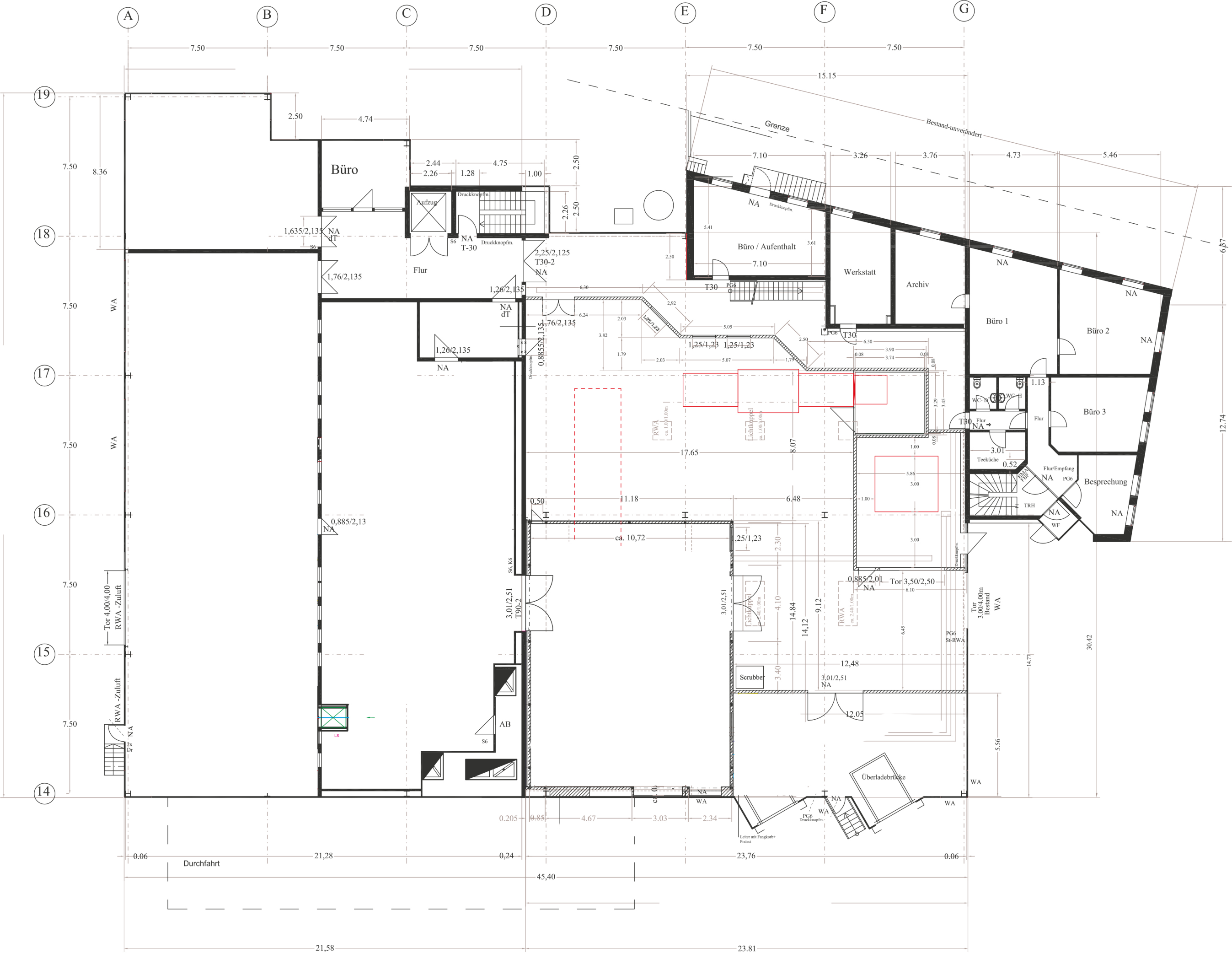
Erdgeschoss
