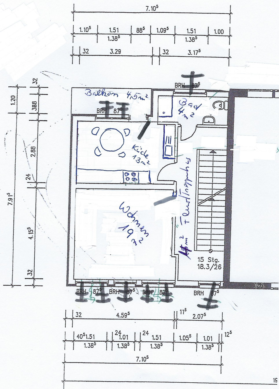
Grundriß OG
