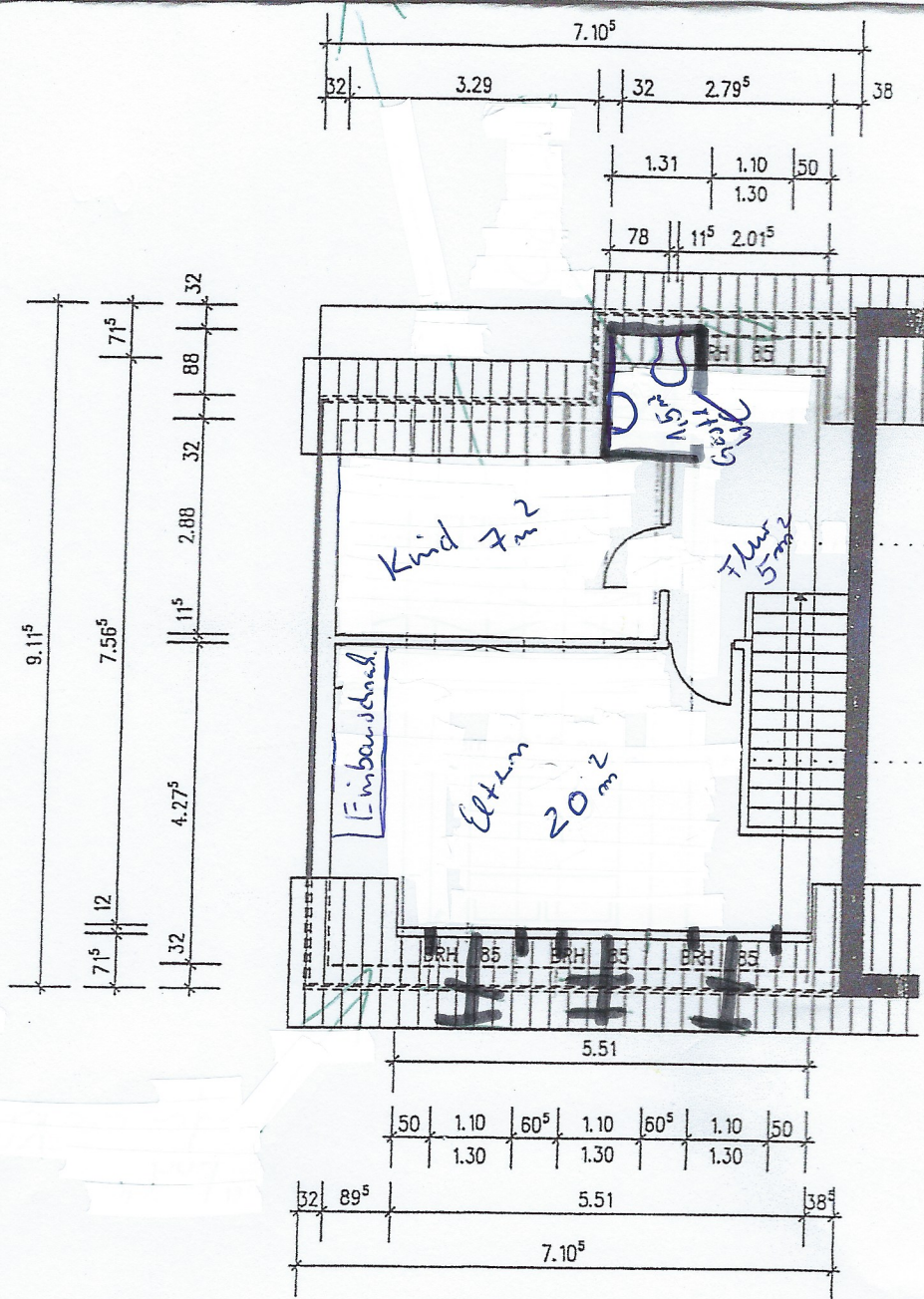
Grundriß DG
