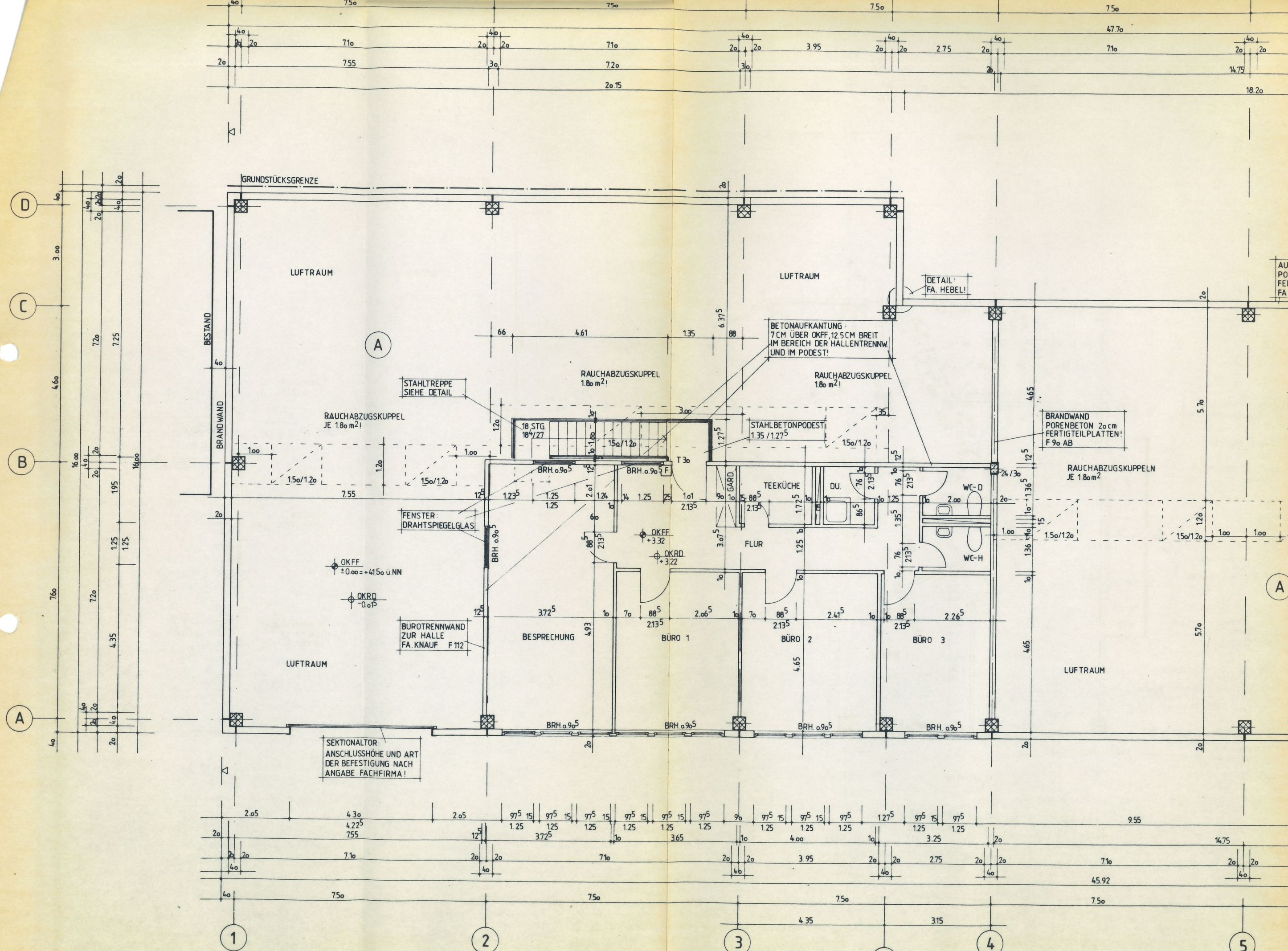
1. OBERGESCHOSS
