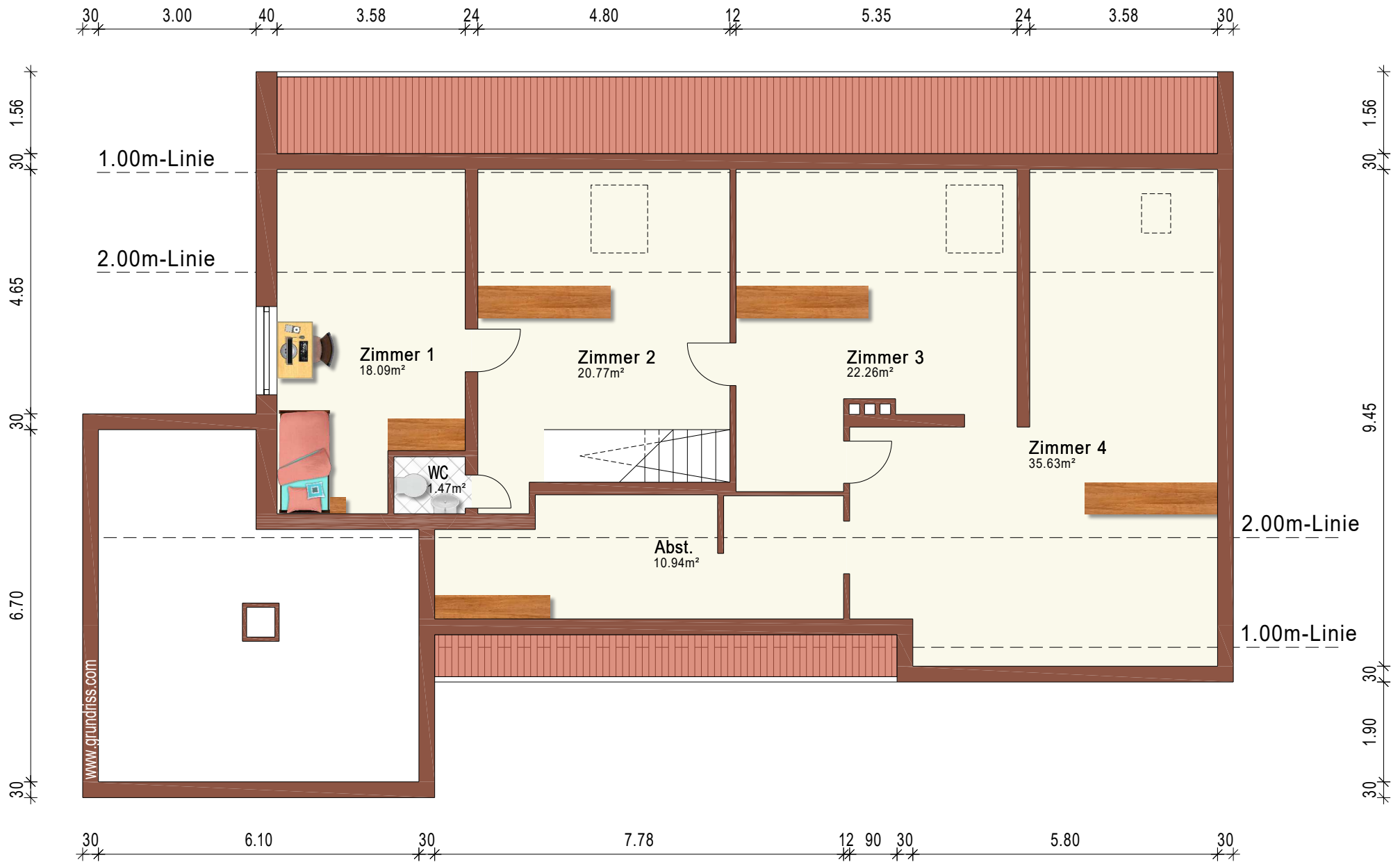
Dachgeschoss
