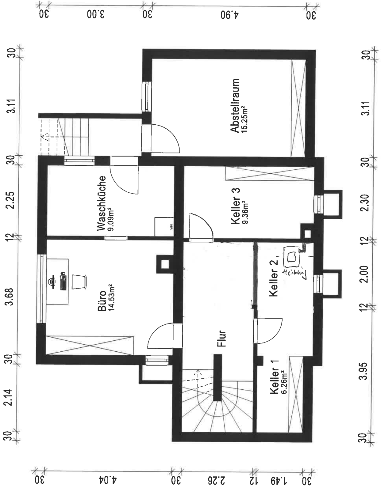
Kellergeschoss
