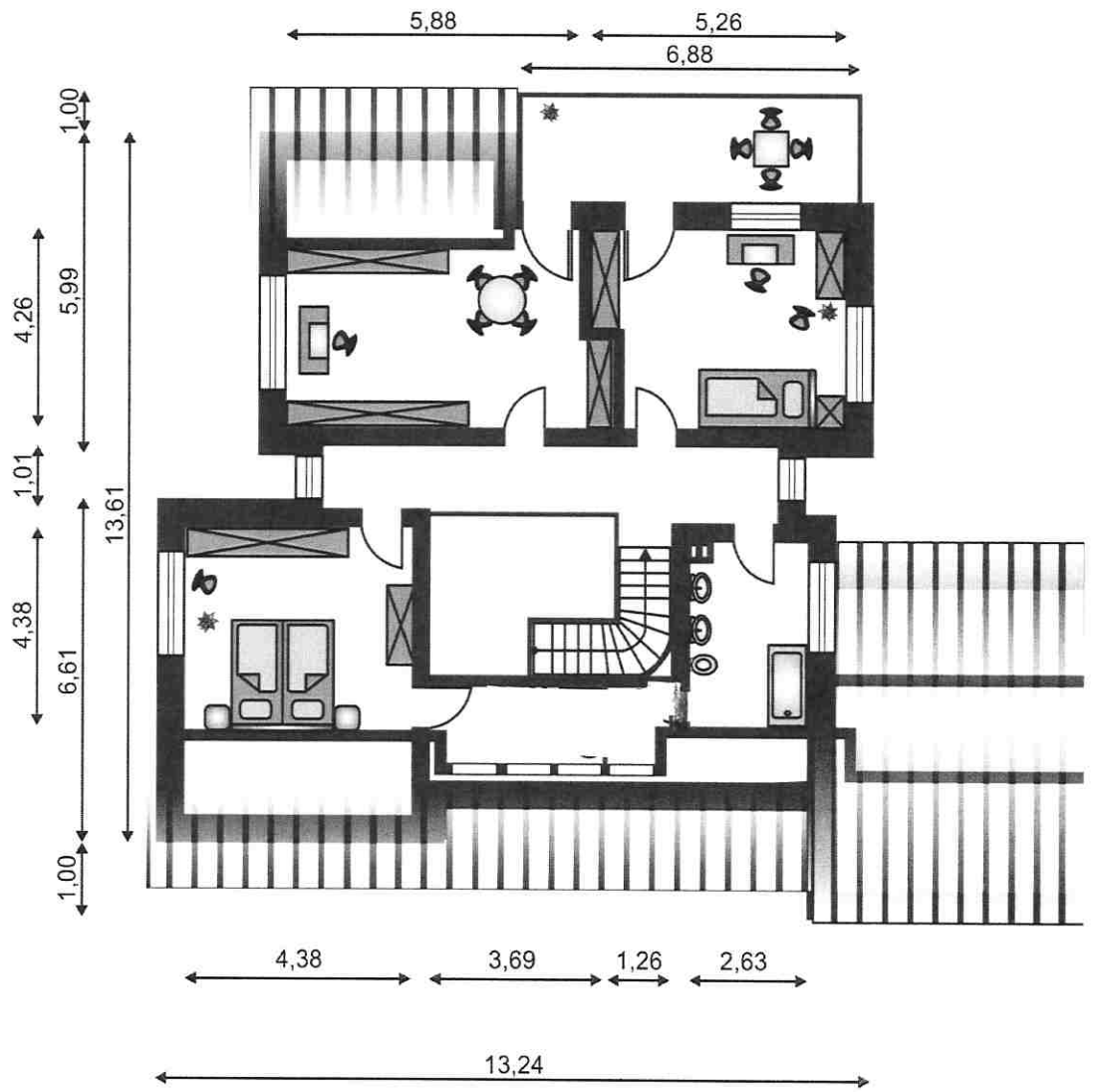
Dachgeschoss
