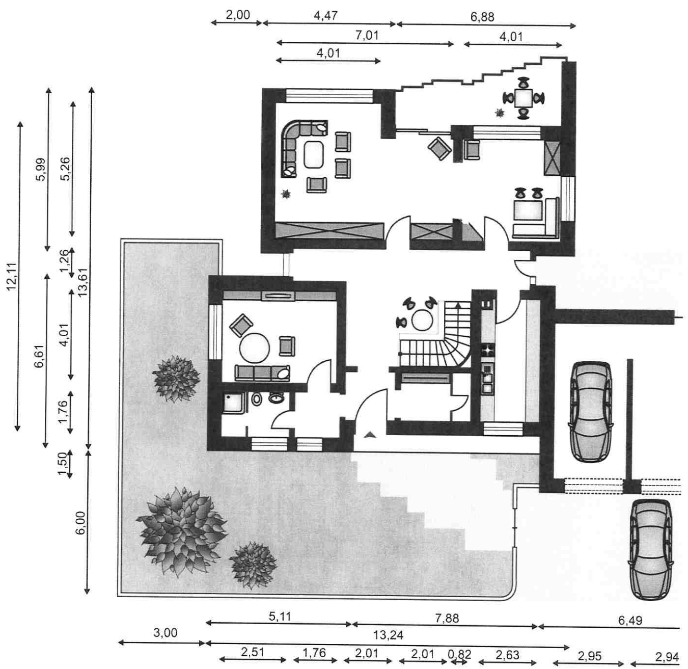
Erdgeschoss
