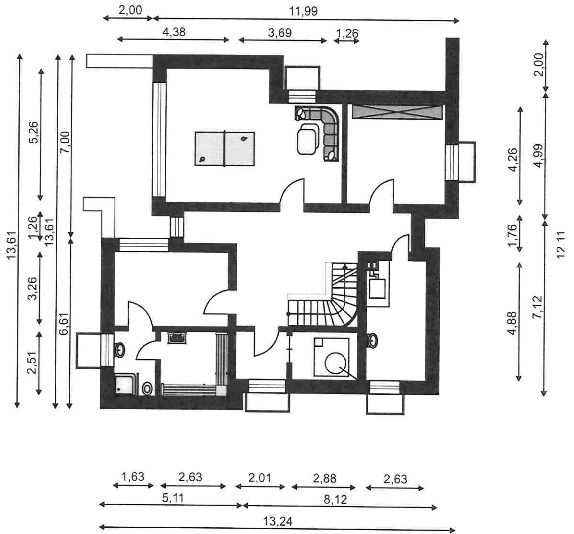
Kellergeschoss
