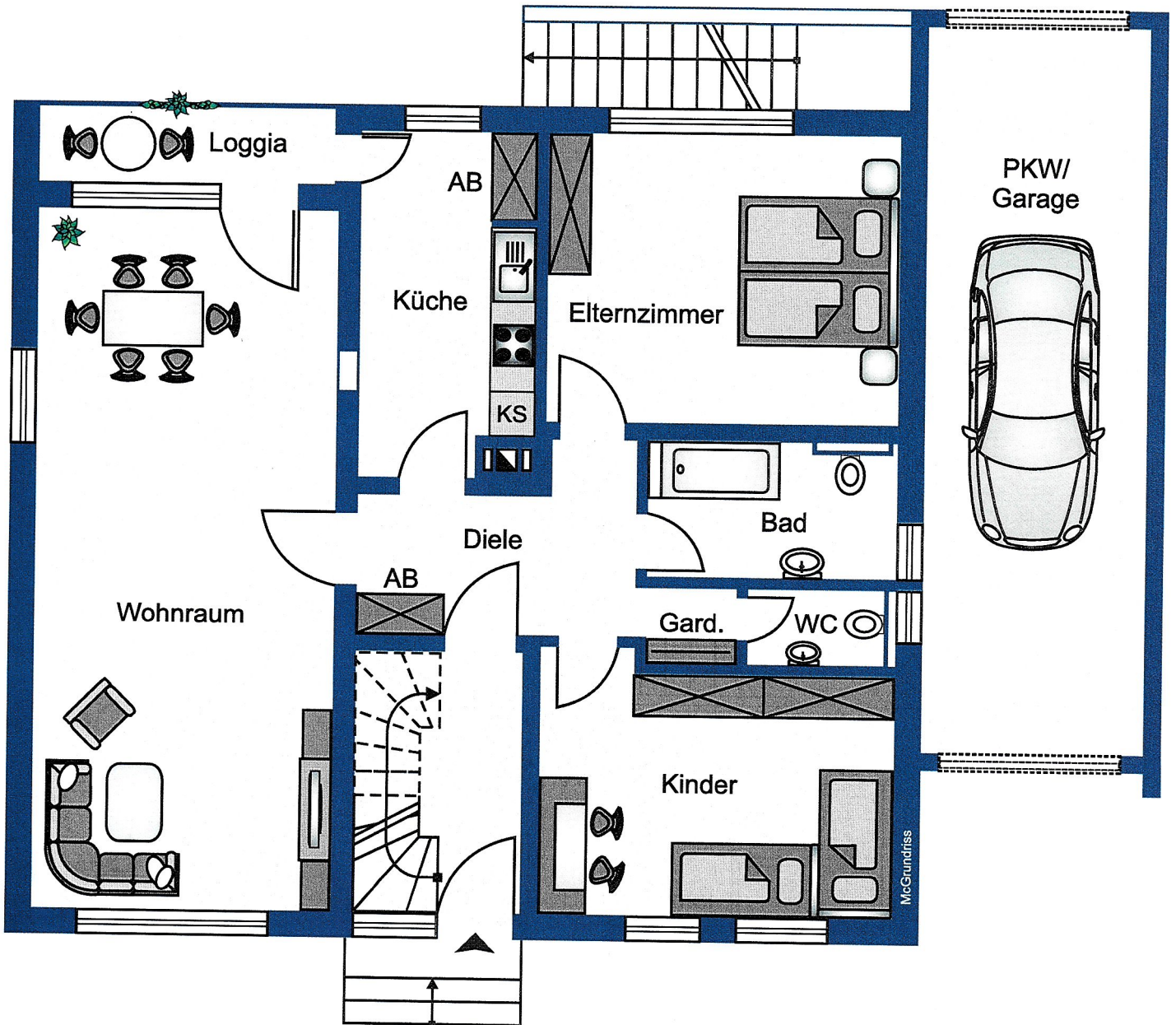
Erdgeschoss
