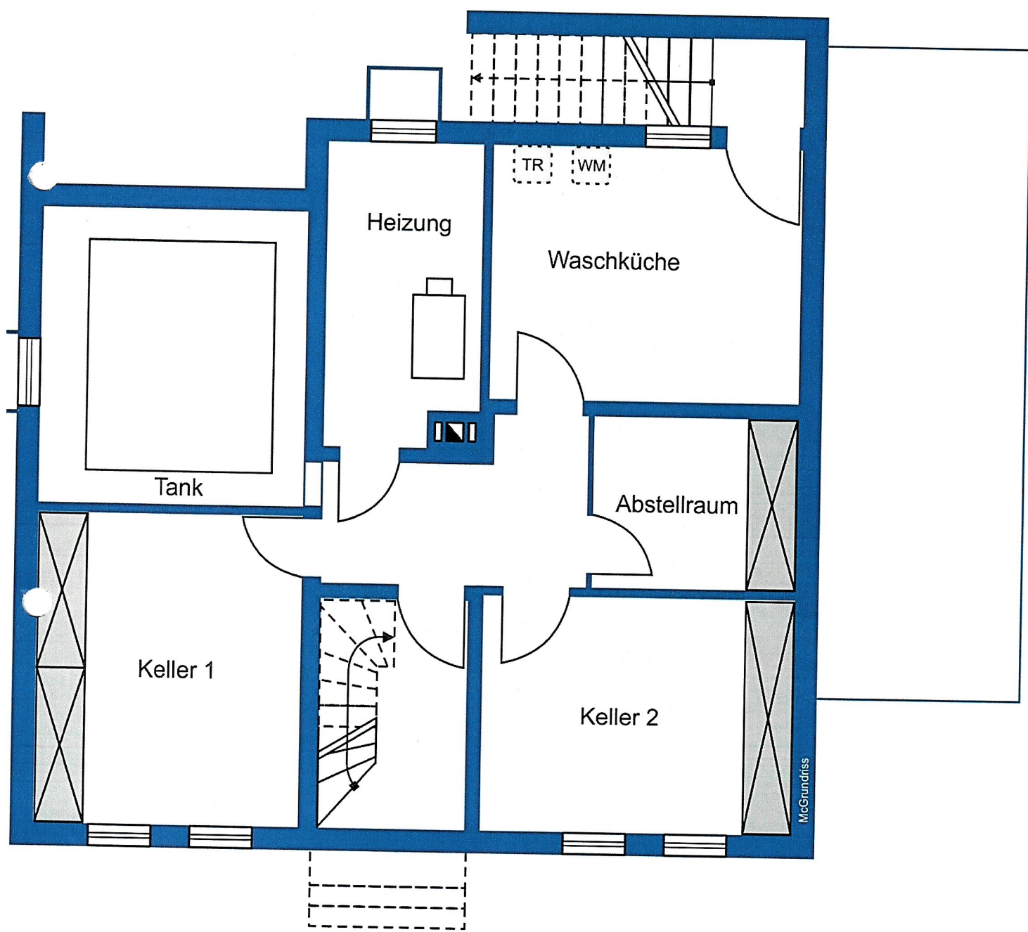
Kellergeschoss
