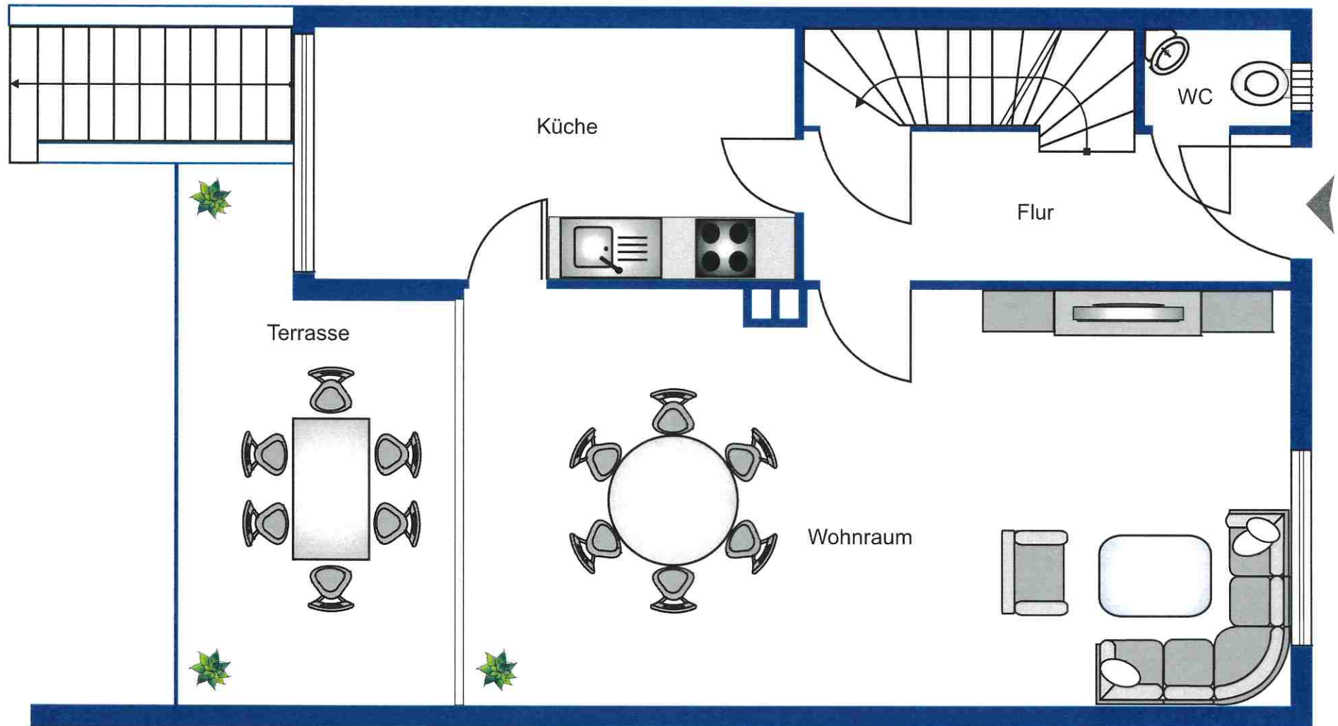
Erdgeschoss
