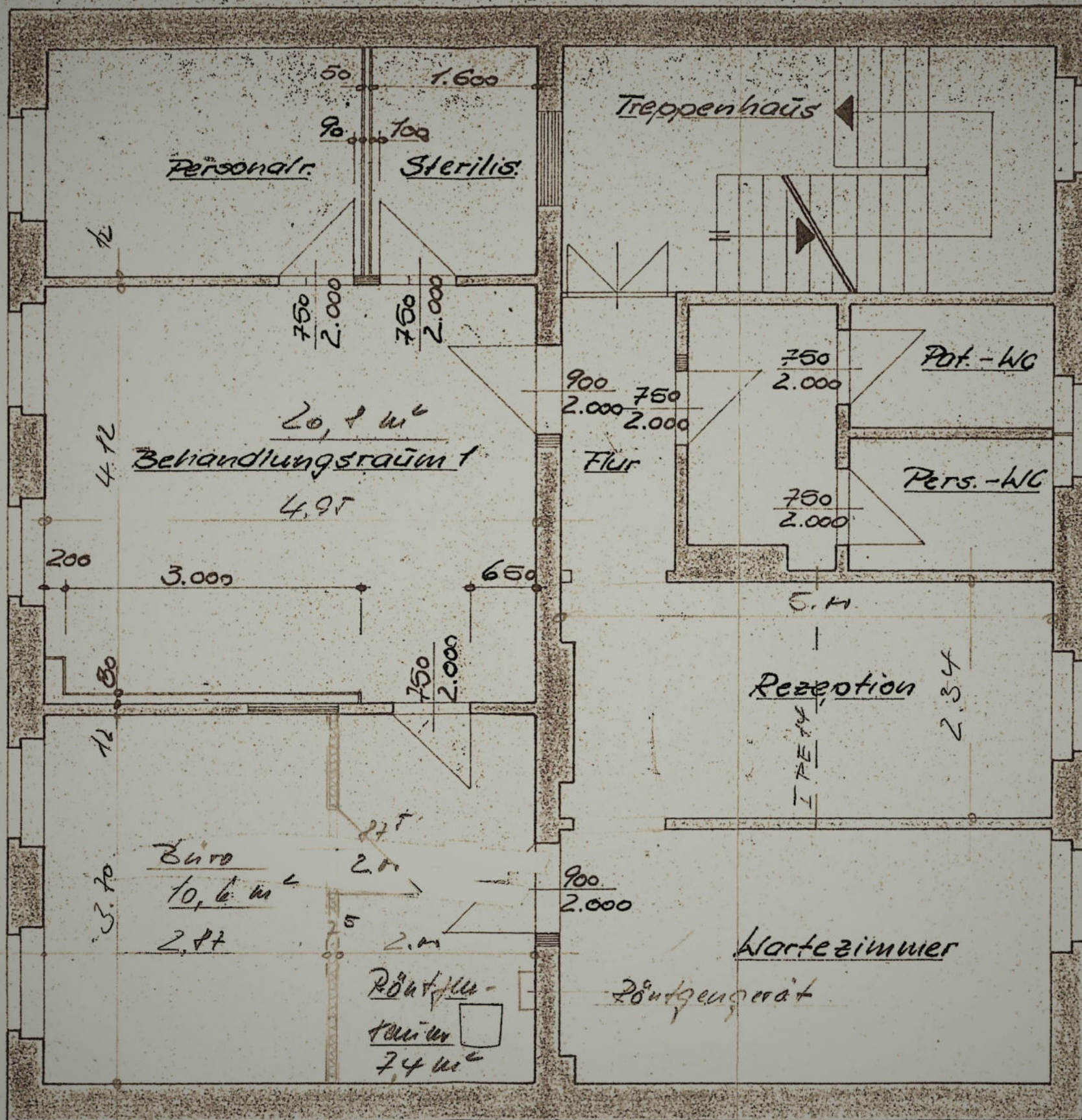
Grundriß 1. Obergeschoß
