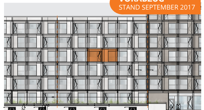
Ansicht Schiffahrtskanal
