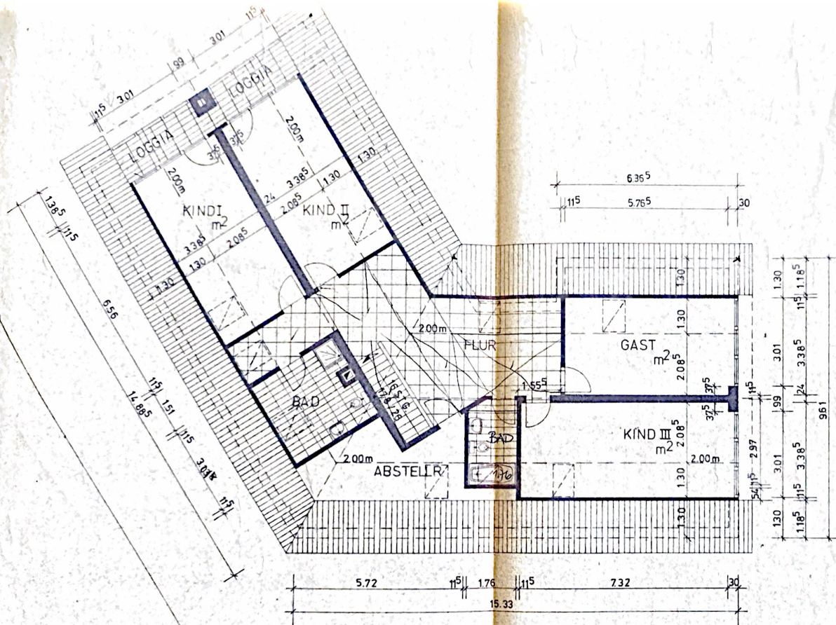
DACHGESCHOSS M. 1:100
