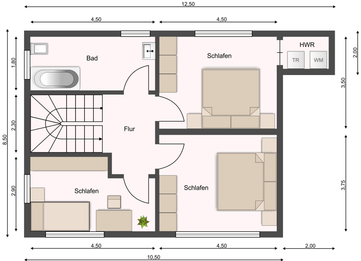
Dachgeschoss Haus West
