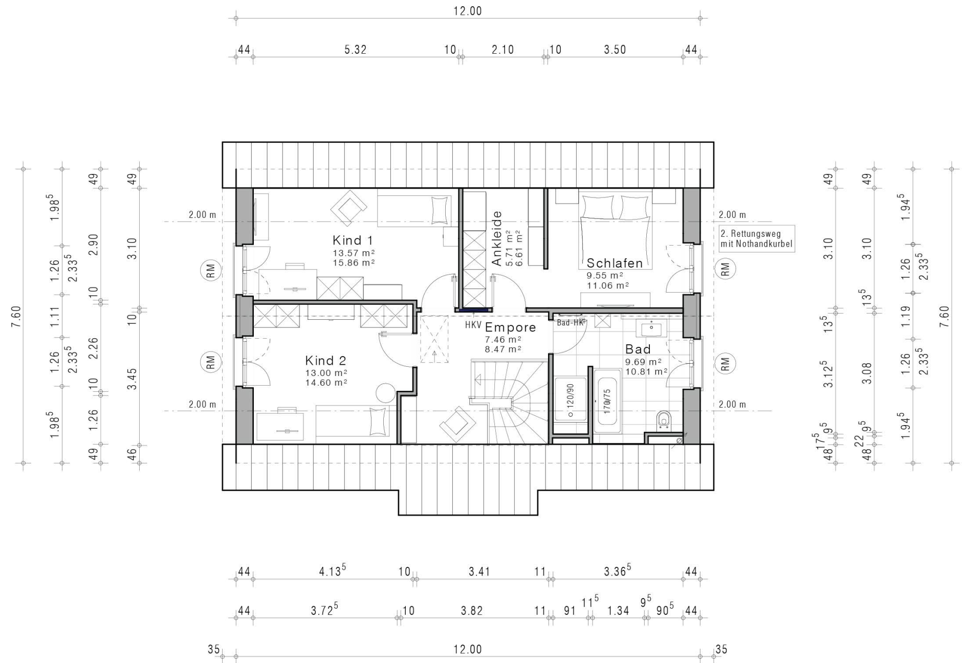
DACHGESCHOSS 58.98 m 2
